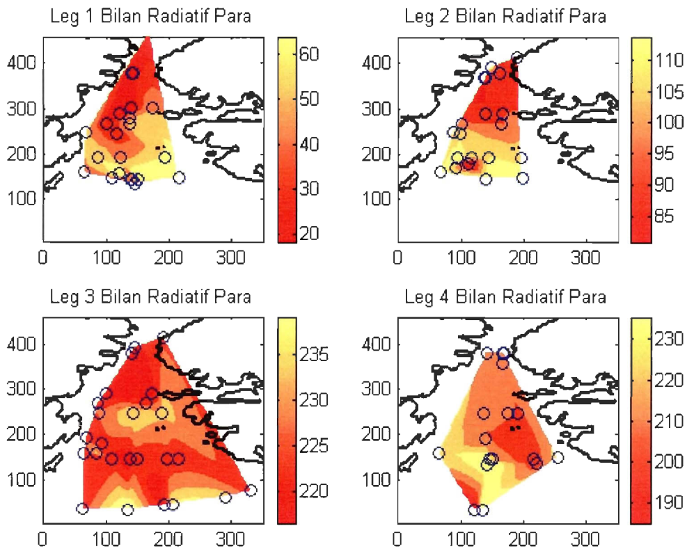
Figure 43 : Bilan radiatif paramétrisé ( \text{W m}^{-2} ) provenant du modèle glace/neige pour chacun des legs. Notez les différences d'échelles. Coordonnées MTU.
