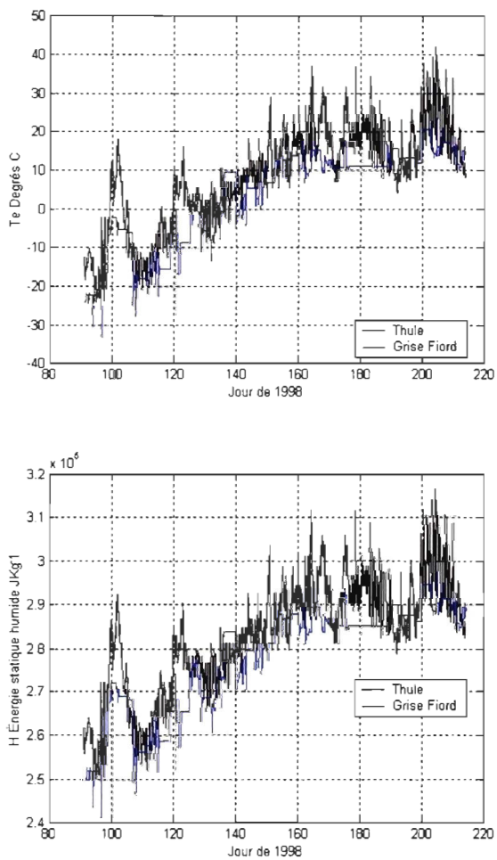
Figure 24 : Température équivalente T_e en degrés °C et énergie statique humide H en 10^5 \text{ J kg}^{-1} pour Thule et Grise Fjord.
