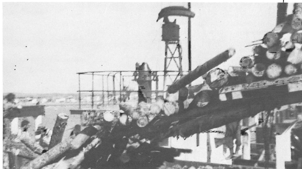
Bois de pulpe versé directement de la benne du camion à la goélette au quai de Rimouski. Cette façon de procéder endommageait toutefois la goélette.
