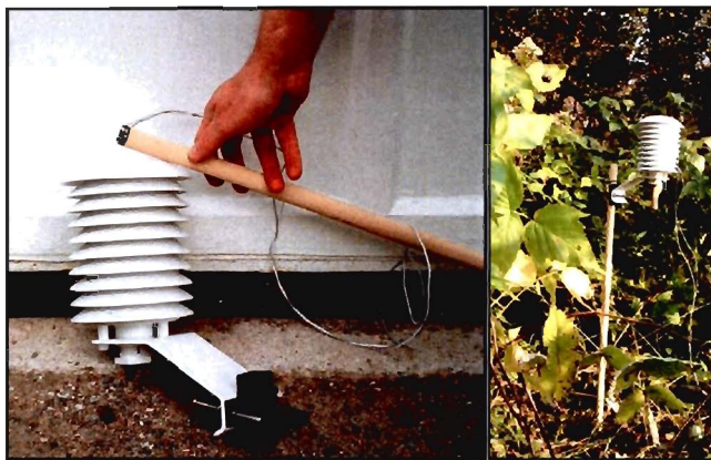
Figure 2.1. Capteur de température iButton et abris anti-rayonnement implantés à la station 1 à Ragueneau.
