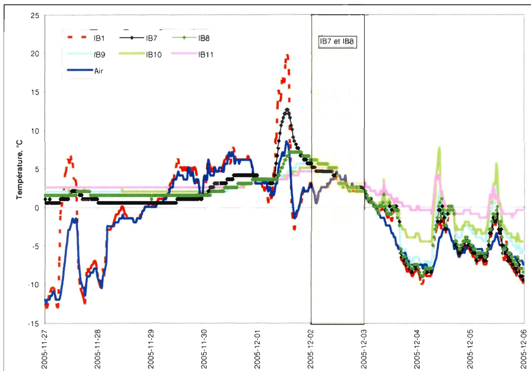
Figure A.8. Signature thermique du recul du 2 décembre 2005 impliquant les iB7 et iB8 de l'unité de silt marin à la station 3.
