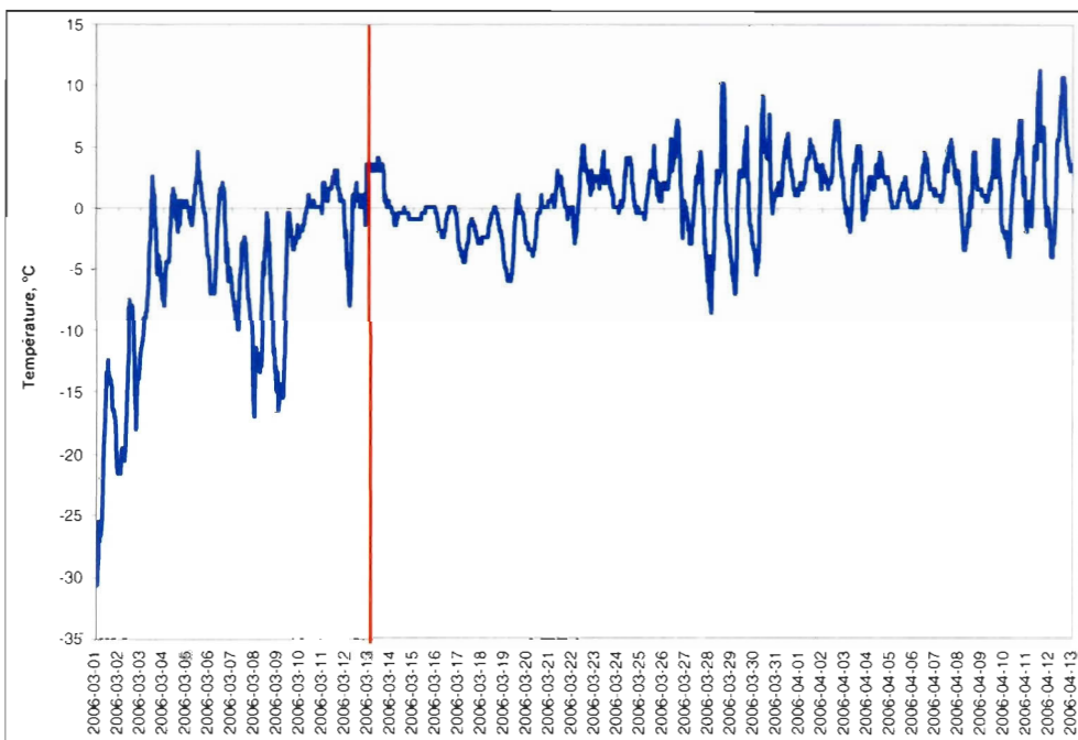
Figure 5.3. Identification de la fin du régime de températures froides et du début du dégel printanier de la saison 2005-2006 le 13 mars 2006 à Ragueneau.
