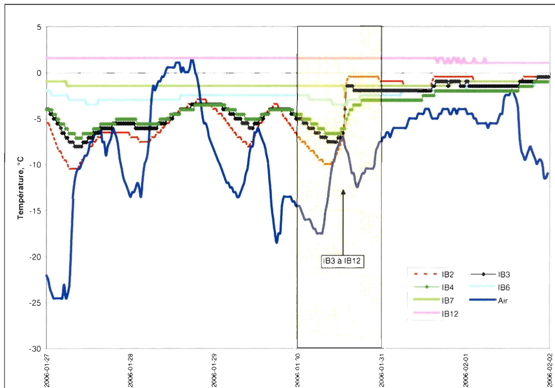
Figure A.9. Signature thermique de la perturbation du 30 janvier 2006 impliquant toute la tige de l'unité de silt marin à la station 1.
