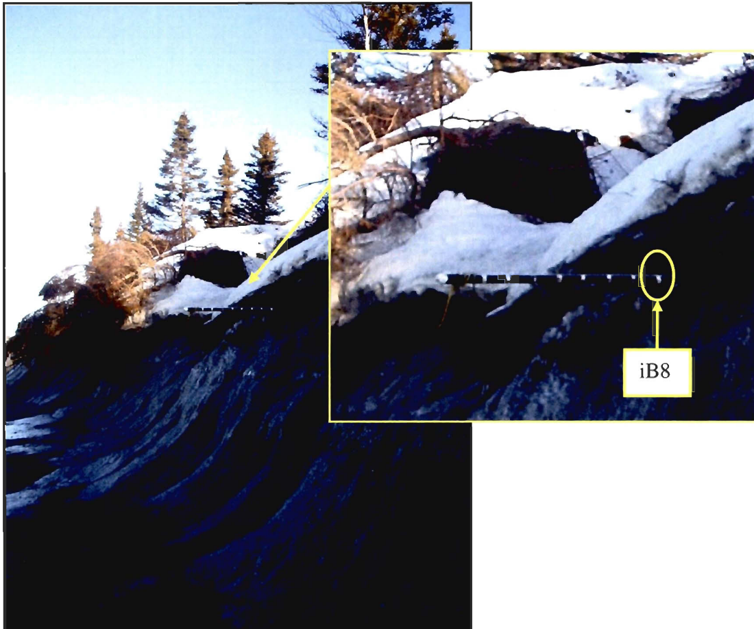
Figure A.14. État de la falaise et position des iButtons le 30 mars 2006 dans l'unité de silt de la station 2.
