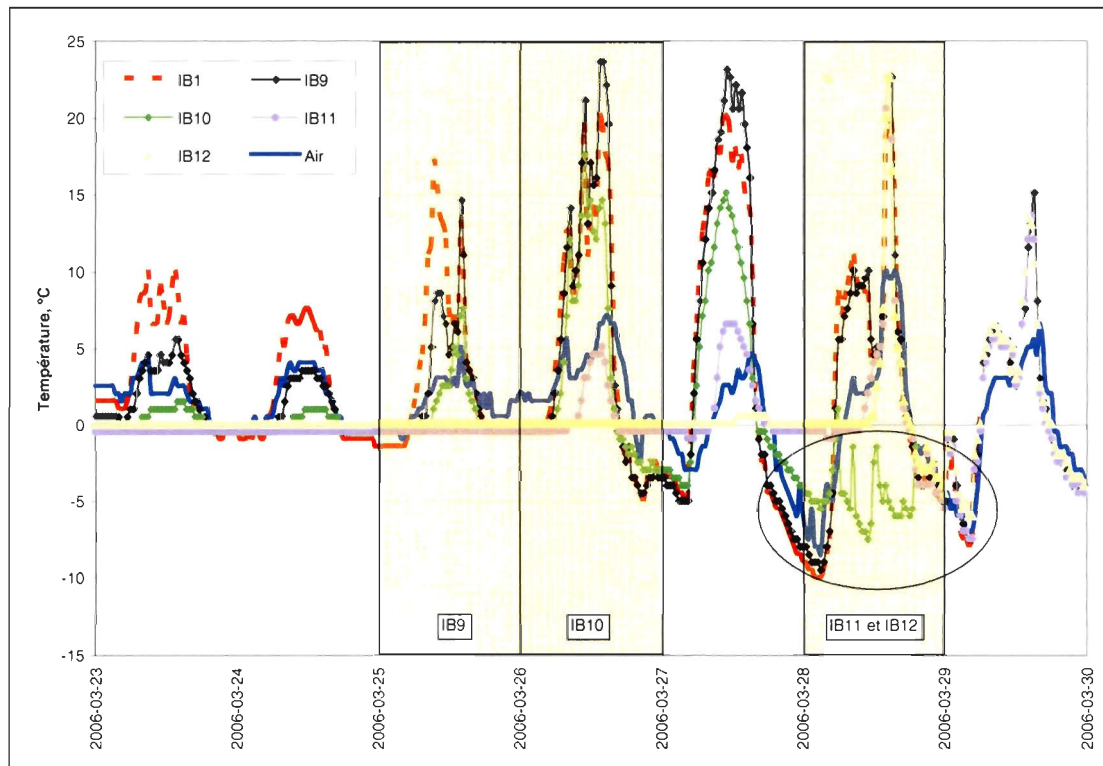
Figure A.15. Signature thermique des reculs du 25, 26 et 28 mars 2006 impliquant les iB9 à iB12 de l'unité de silt marin à la station 3.
