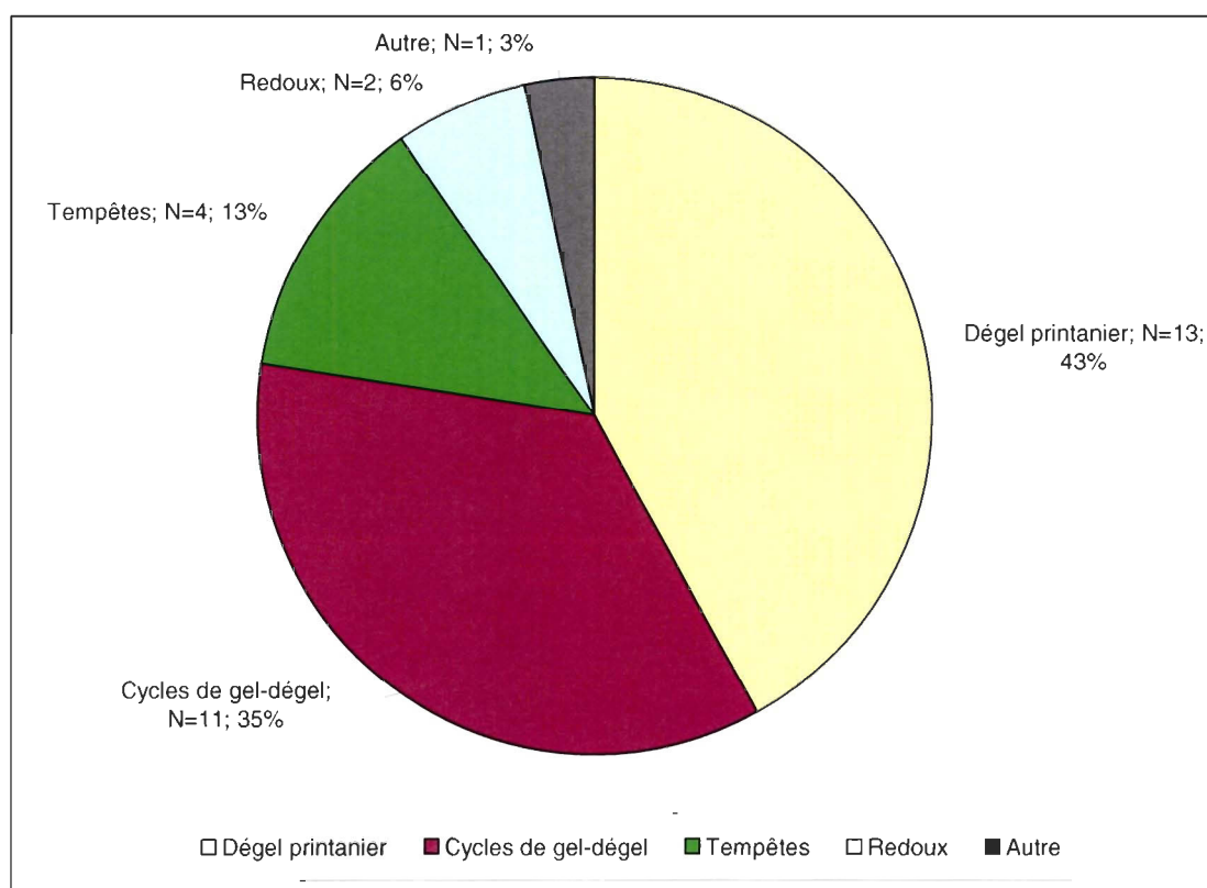
Figure 5.8. Part relative des grandes situations climatiques ayant générés des reculs dans les falaises à Ragueneau.
