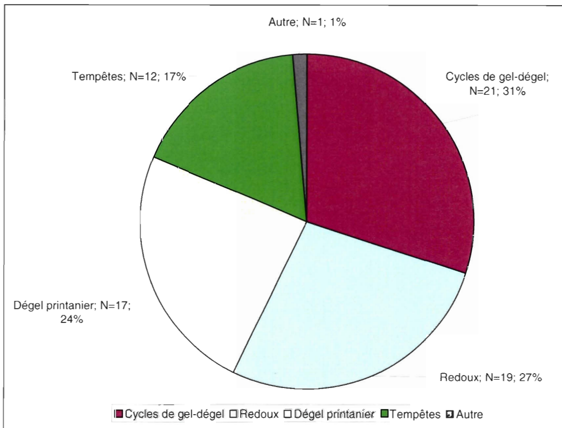
Figure 5.9. Part relative du nombre de iButtons impliqués dans les reculs des falaises en fonction des grandes situations climatiques à Ragueneau.
