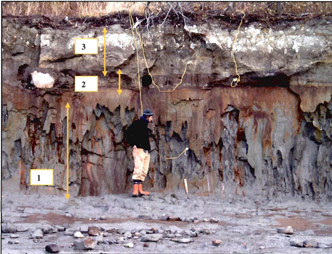
Figure 3.4. Stratigraphie à la station 1 : 1) silt marin; 2) sable intertidal; 3) silt intertidal.
