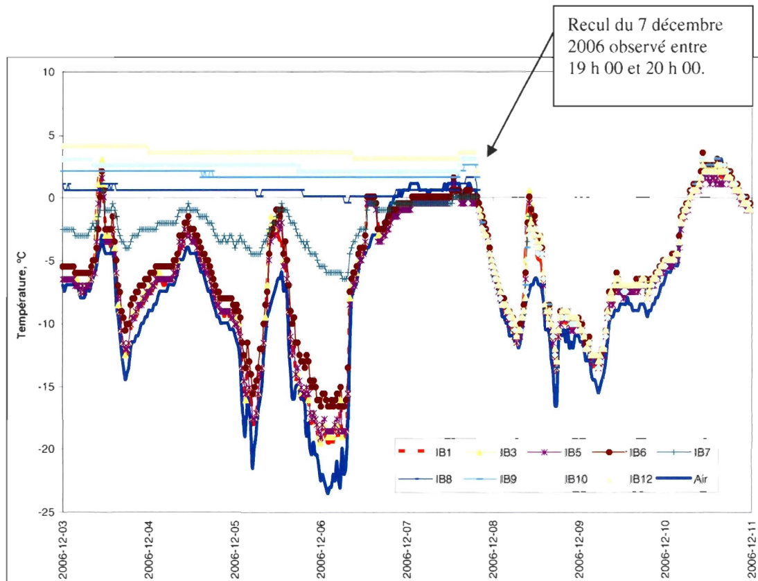
Figure 2.5. Principe de la méthode d'analyse des évènements de recul à l'aide du régime thermique : exemple de l'évènement de recul du 7 décembre 2006.
