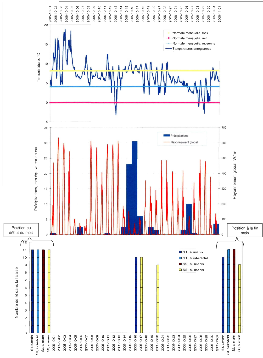
Figure 4.1. Conditions climatiques et reculs des falaises observés au mois d'octobre 2005 à Ragueneau.
