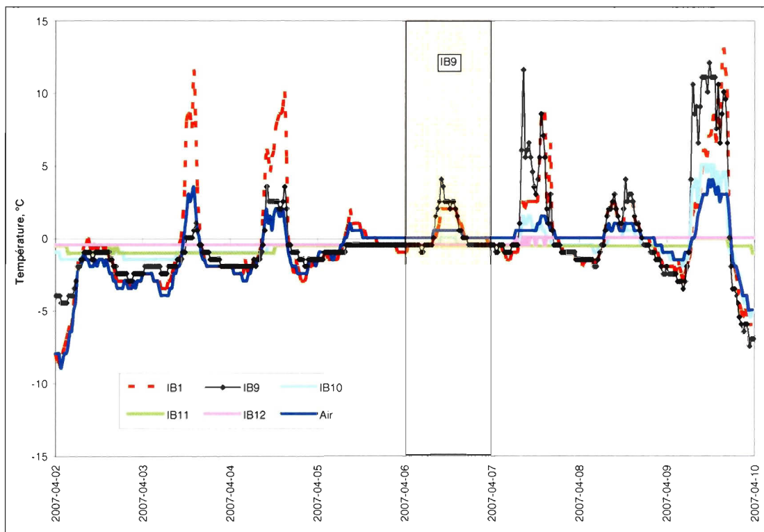
Figure A.36. Signature thermique du recul du 6 avril 2007 impliquant le iB9 de l'unité de silt marin à la station 2.
