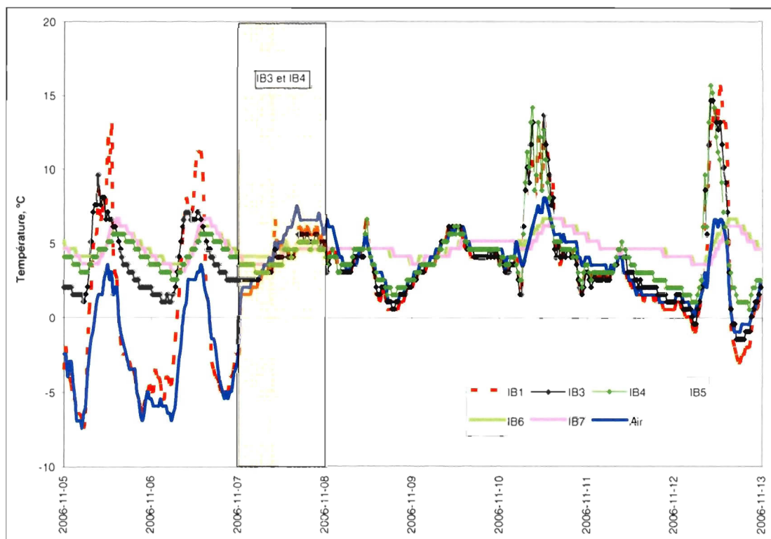
Figure A.23. Signature thermique du recul du 7 novembre 2006 impliquant le iB3 et le iB4 de l'unité de silt marin à la station 3.
