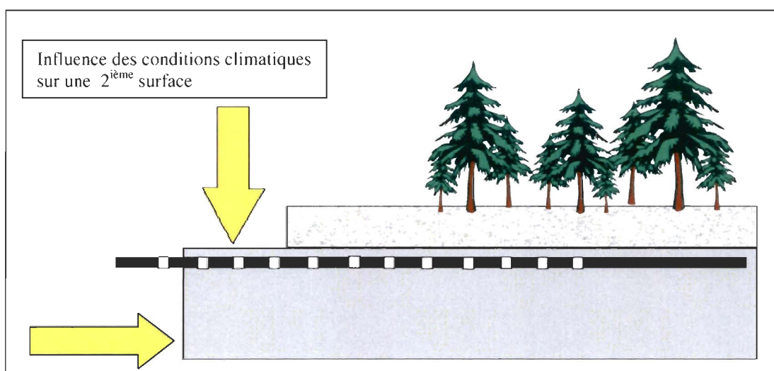
Figure.4.29. Schéma du développement d'un plateau à la suite du recul de l'unité supérieure permettant aux conditions climatiques d'influencer les comportements thermiques des iButtons depuis une surface supplémentaire (horizontale).
