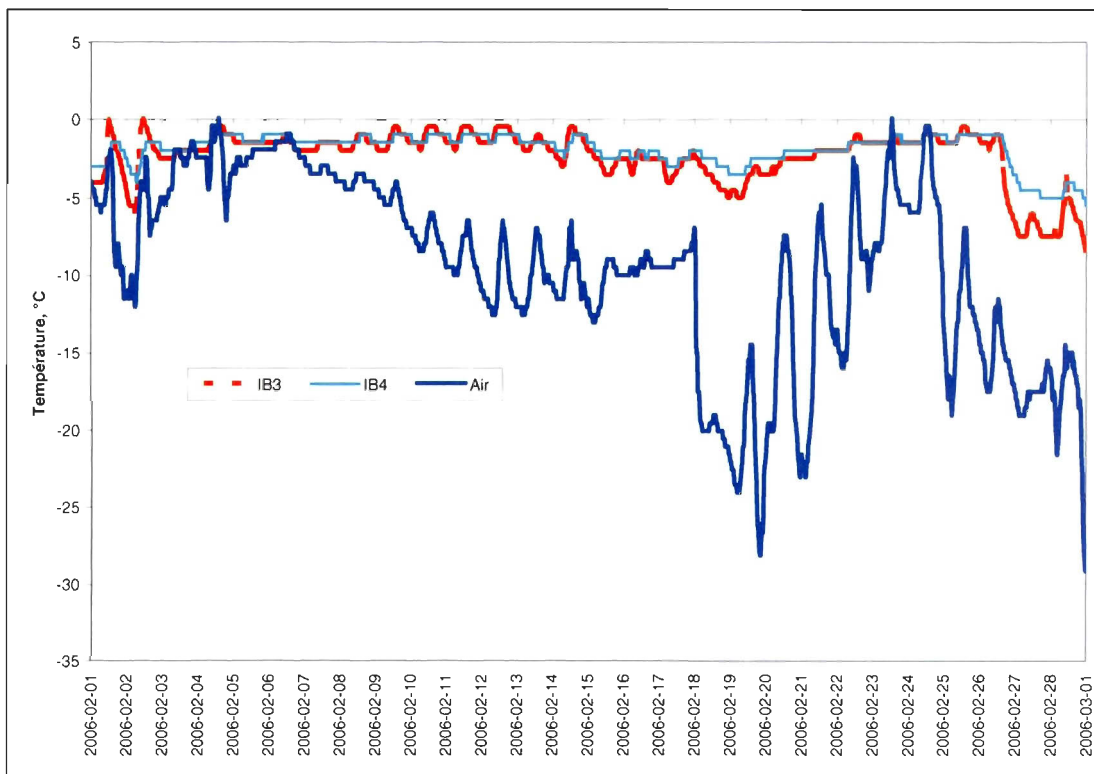
Figure 4.9. Effet du couvert de neige sur les températures des iB3 et iB4 à la station 2 et fusion partielle à la suite des conditions du 25 et 26 février 2006.
