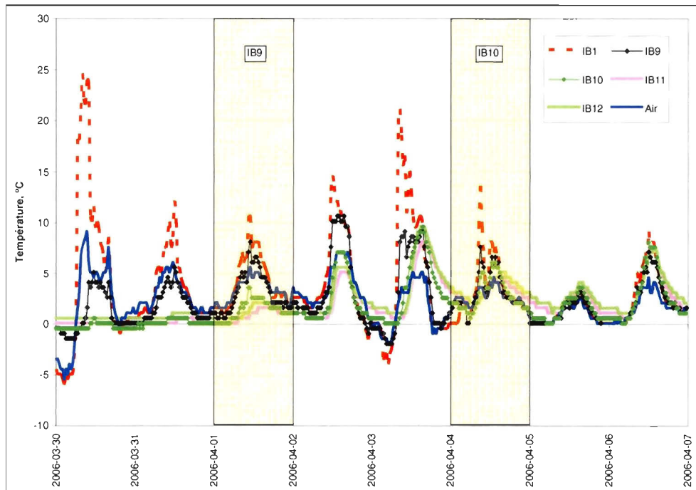
Figure A.17. Signature thermique du recul du 1 er et du 4 avril 2006 impliquant les iB9 et iB10 de l'unité de silt marin à la station 2.
