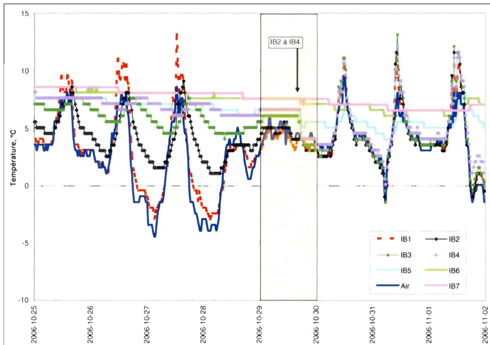
Figure A.21. Signature thermique du recul du 29 octobre 2006 (18 h 00) impliquant les iB2 à iB4 de l'unité de silt marin à la station 1.
