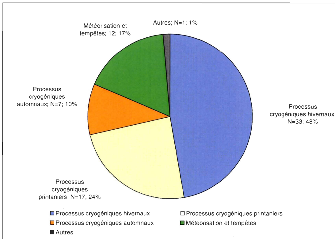
Figure 5.26. Quantification des processus responsables de l'érosion des falaises de silt marin à Ragueneau.
