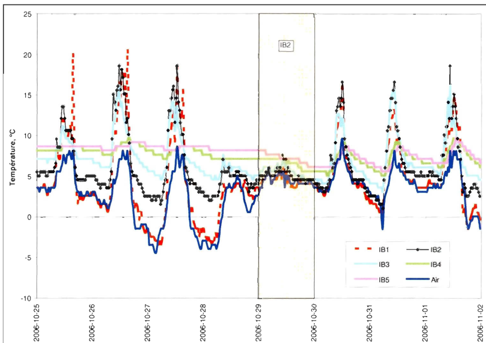
Figure A.22. Signature thermique du recul du 29 octobre 2006 impliquant le iB2 de l'unité de silt marin à la station 3.
