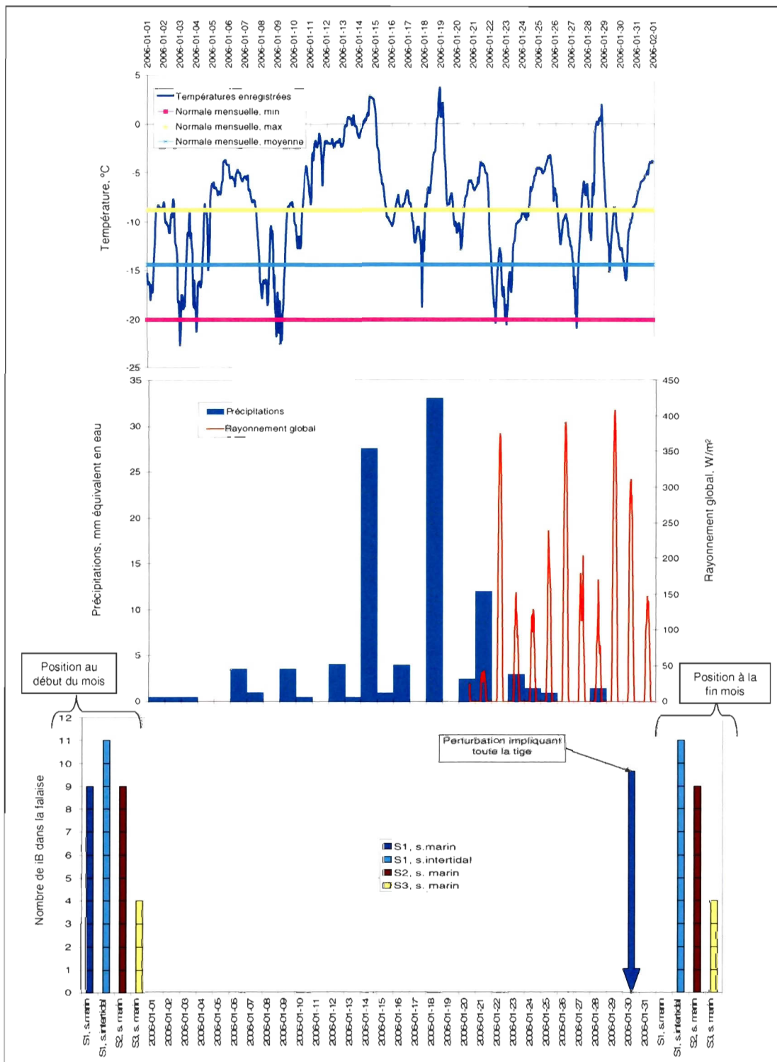
Figure 4.5. Conditions climatiques et reculs des falaises observés au mois de janvier 2006 à Ragneau.
