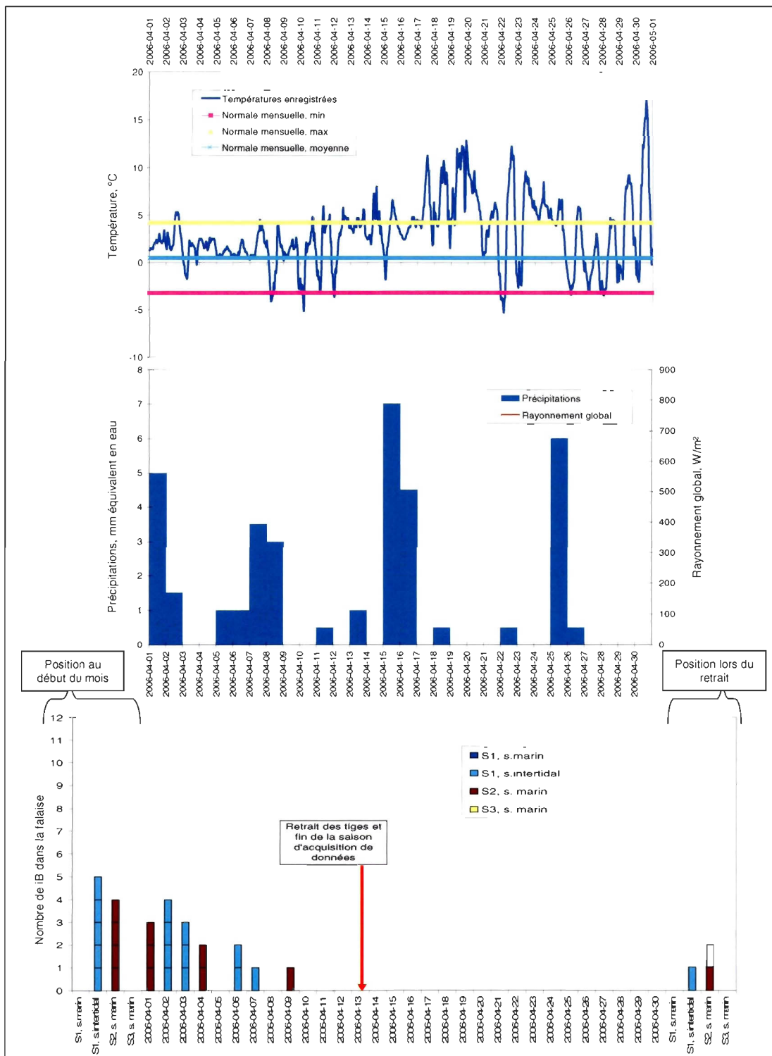
Figure 4.12. Conditions climatiques et reculs des falaises observés au mois d'avril 2006 à Ragueneau.
