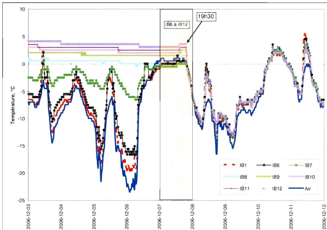
Figure A.27. Signature thermique du recul du 7 décembre 2006 (vers 19 h 30) impliquant les iB6 à iB12 de l'unité de silt marin à la station 1.
