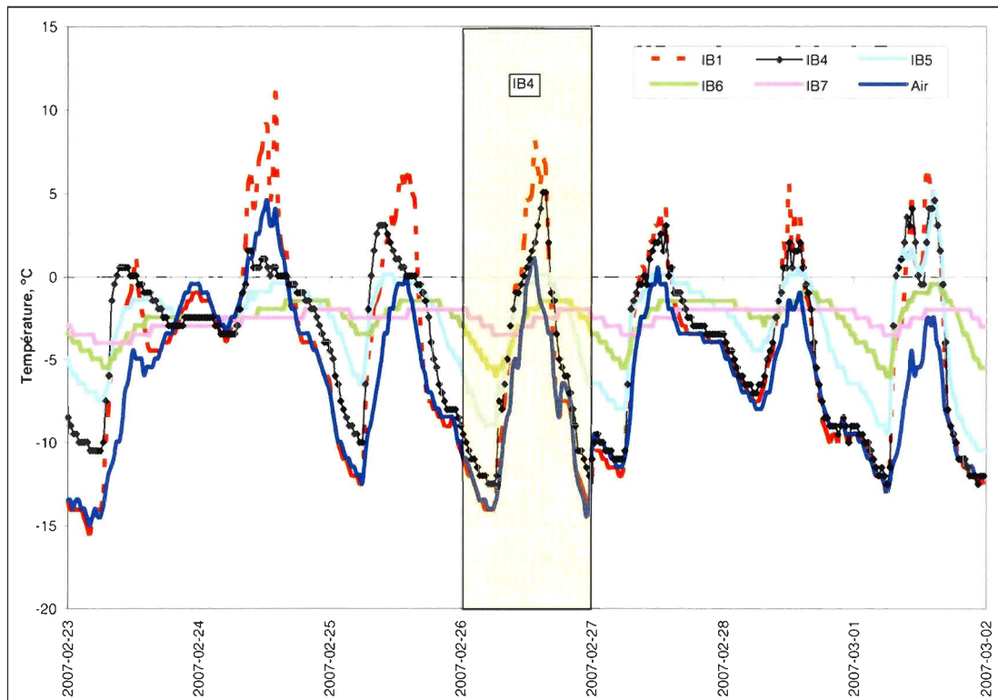
Figure A.30. Signature thermique du recul du 26 février 2007 impliquant le iB4 de l'unité de silt marin à la station 2.
