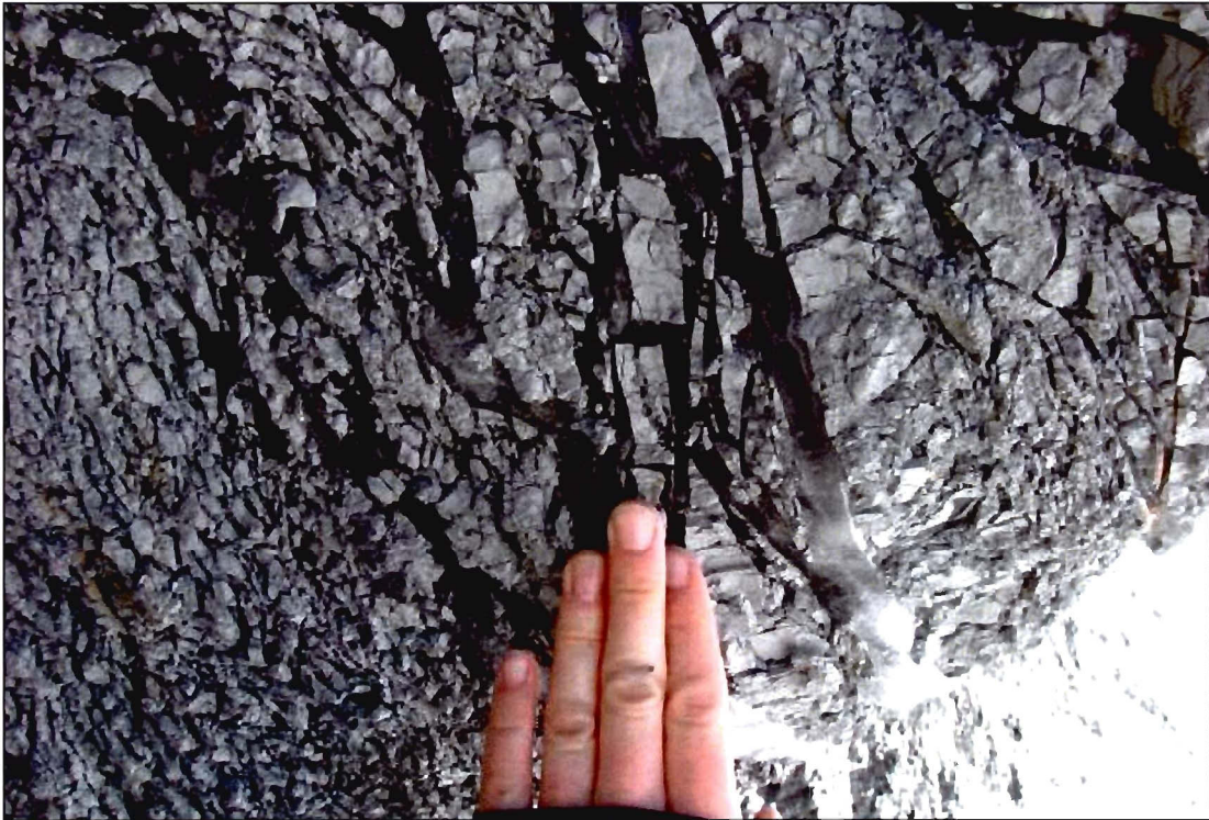
Figure 5.13. Lentilles de glace observé le 9 mars 2007 à Ragueneau
