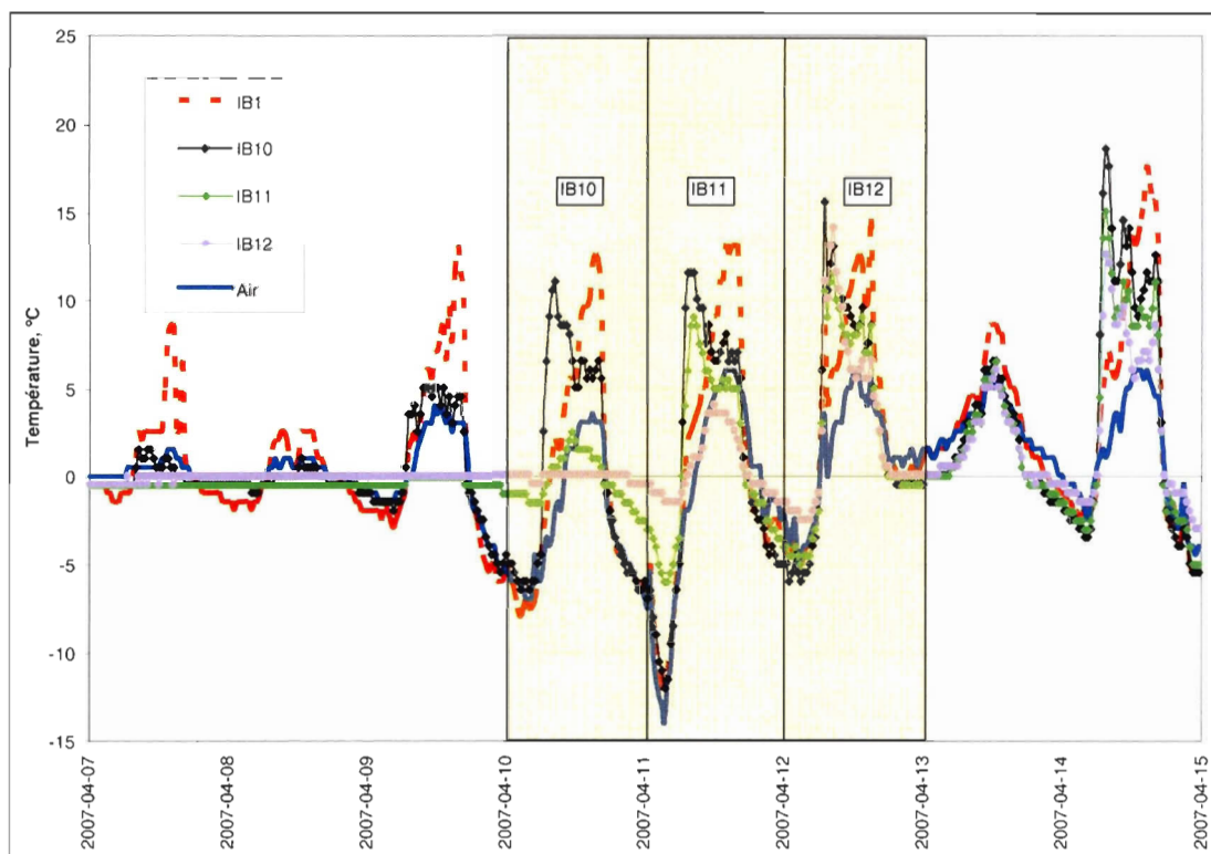
Figure A.37. Signature thermique des reculs du 10, 11 et 12 avril 2007 impliquant les iB10, iB11 et iB12 de l'unité de silt marin à la station 2.
