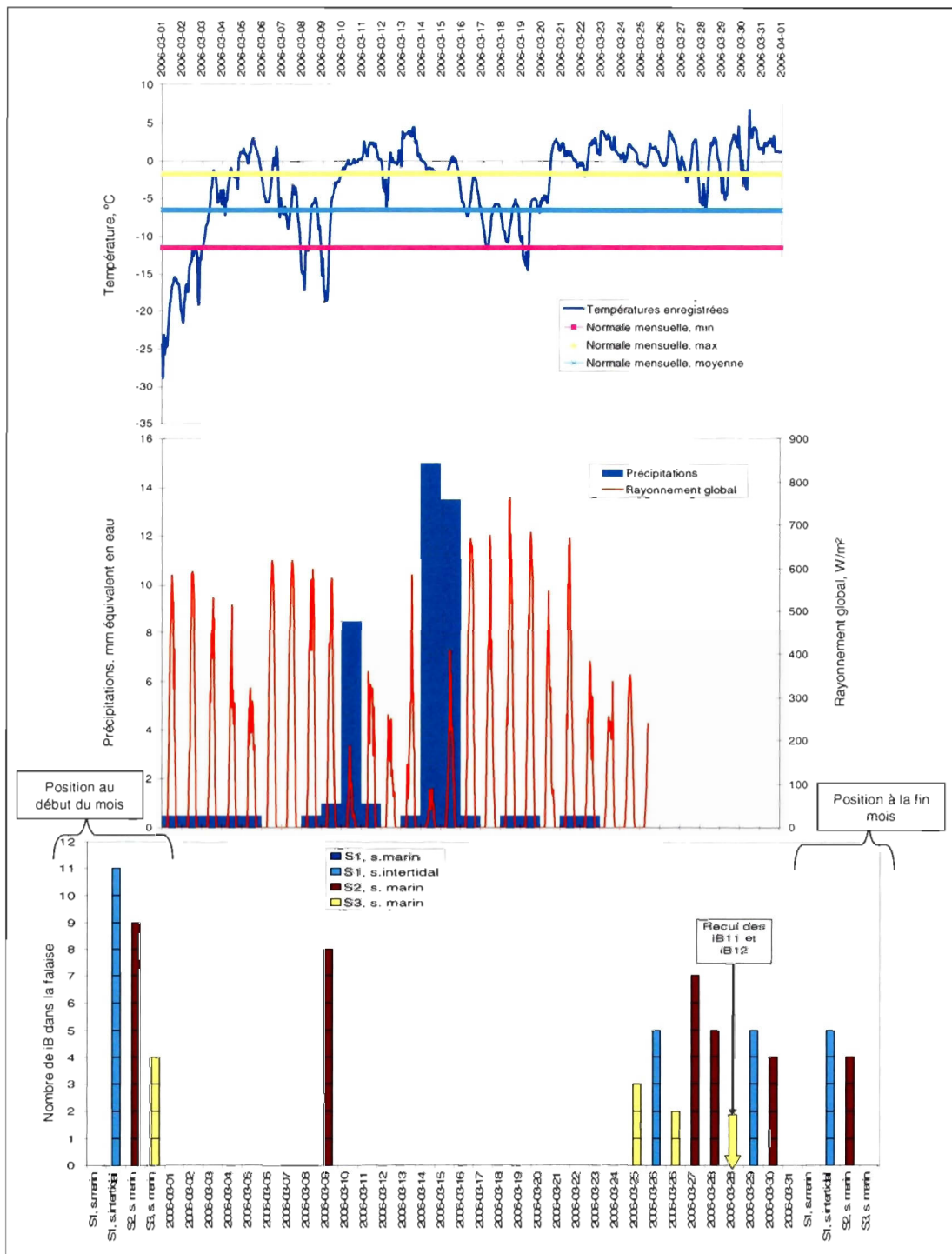
Figure 4.10. Conditions climatiques et reculs des falaises observés au mois de mars 2006 à Ragueneau.
