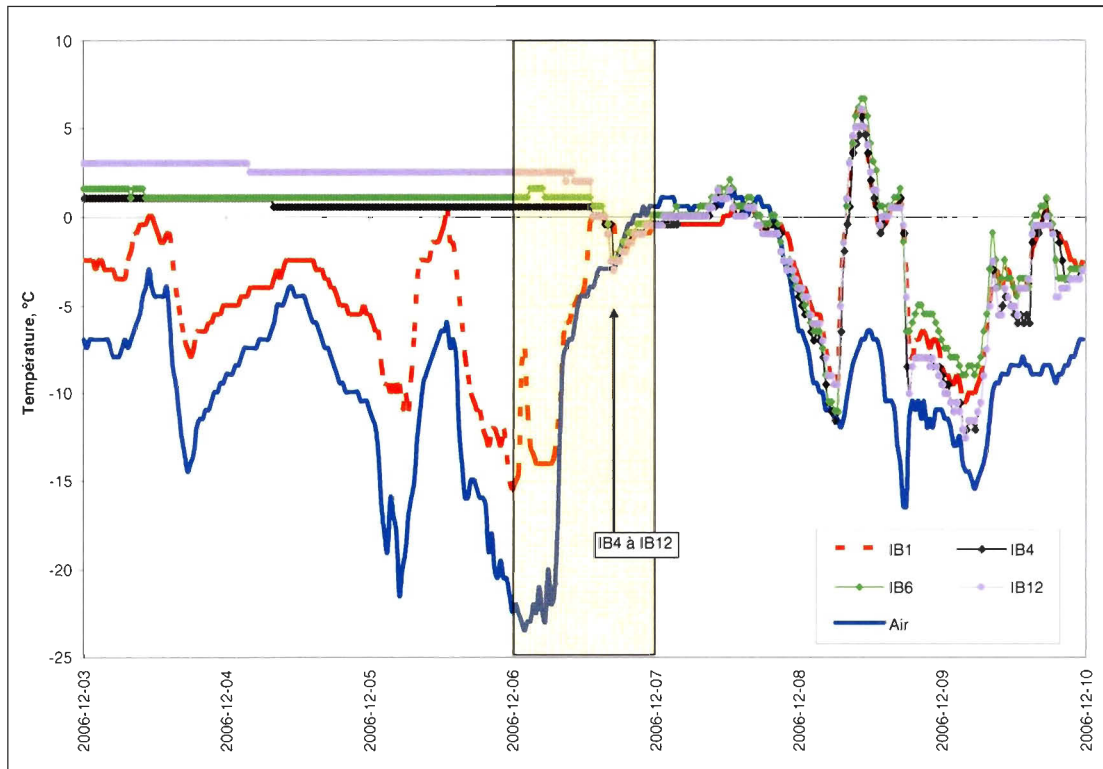
Figure A.26. Signature thermique du recul du 6 décembre (vers 13 h 30) impliquant les iB4 à iB12 de l'unité de silt marin à la station 3.
