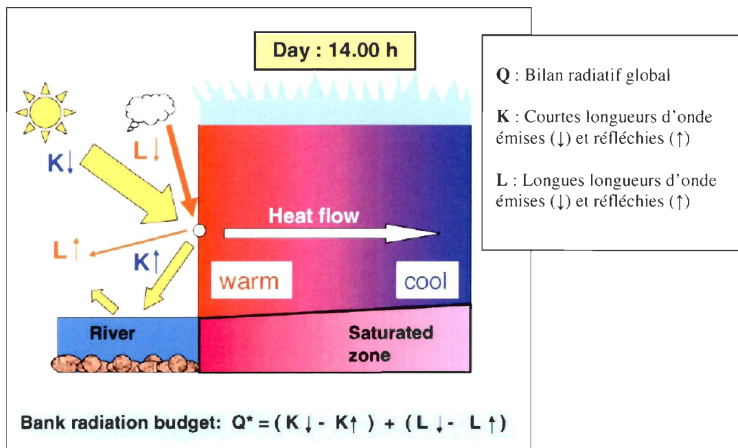
Figure 2.4. Illustration des principes de microclimatologie sur la période diurne
