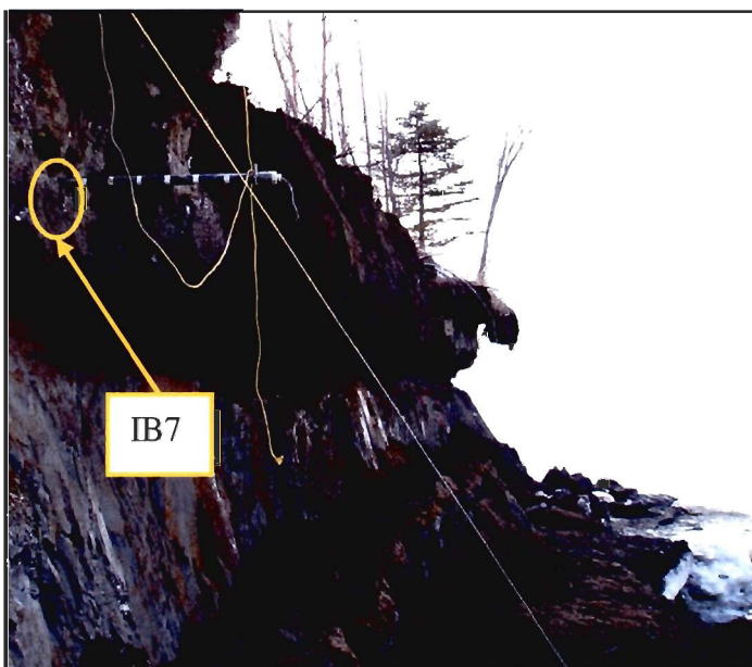
Figure 5.7. État de la falaise de la station 1 et position des iButtons dans l'unité de silt intertidal le 26 mars 2006 (iB7 à peine visible)
