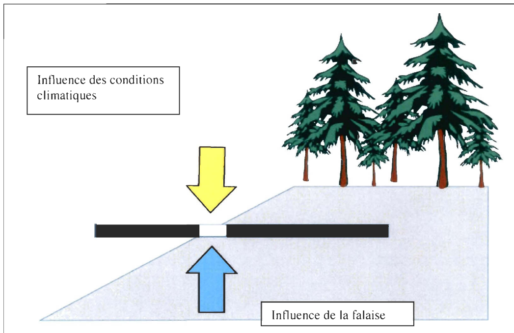
Figure.4.28. Schéma du développement d'une pente douce soulevant des difficultés dans l'analyse des signatures thermiques des iButtons .
