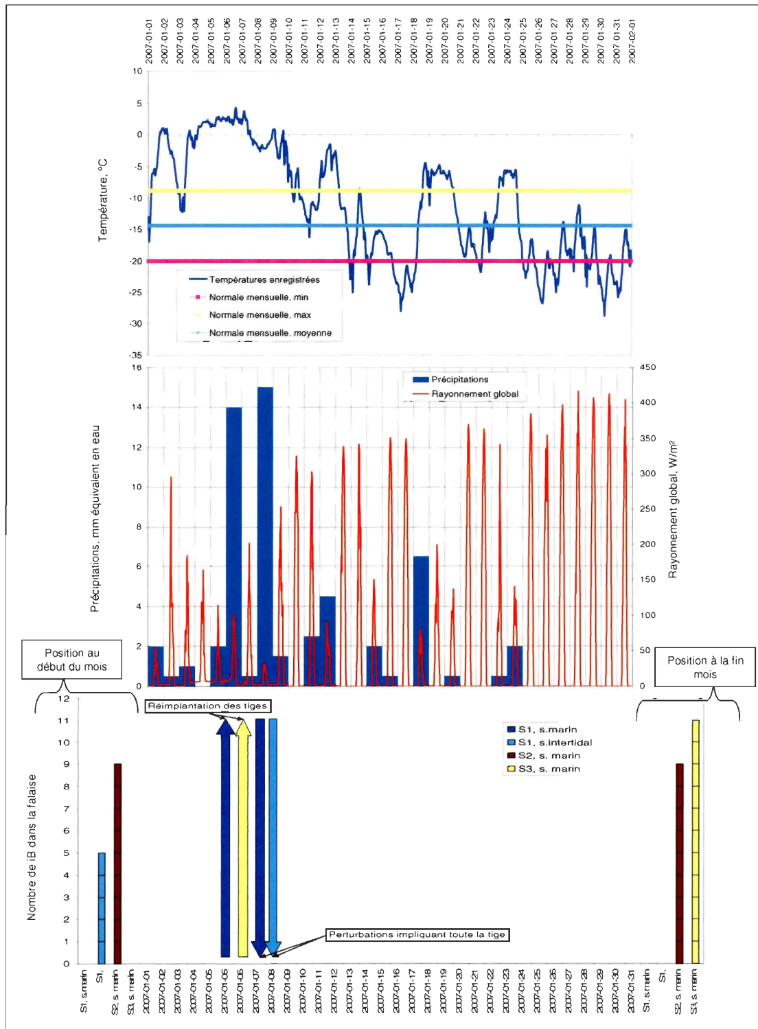
Figure 4.20. Conditions climatiques et reculs des falaises observés au mois de janvier 2007 à Ragueneau.
