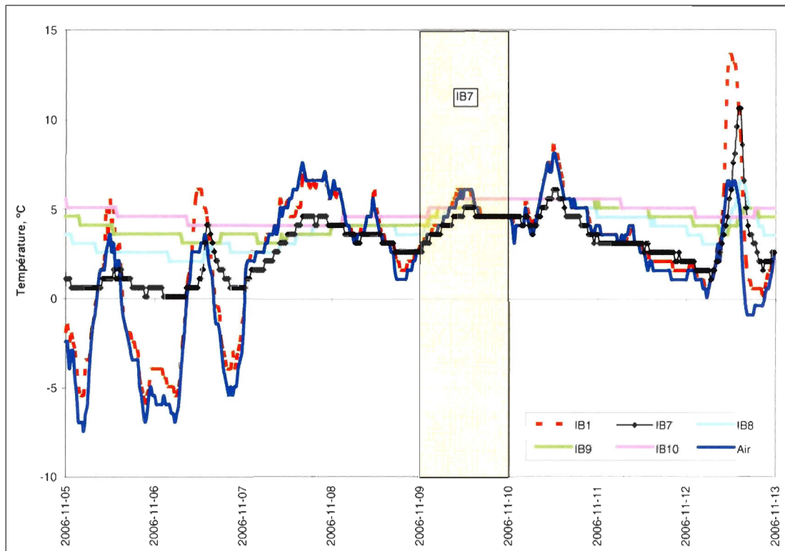
Figure A.24. Signature thermique du recul du 9 novembre 2006 impliquant le iB7 de l'unité de silt intertidal à la station 1.
