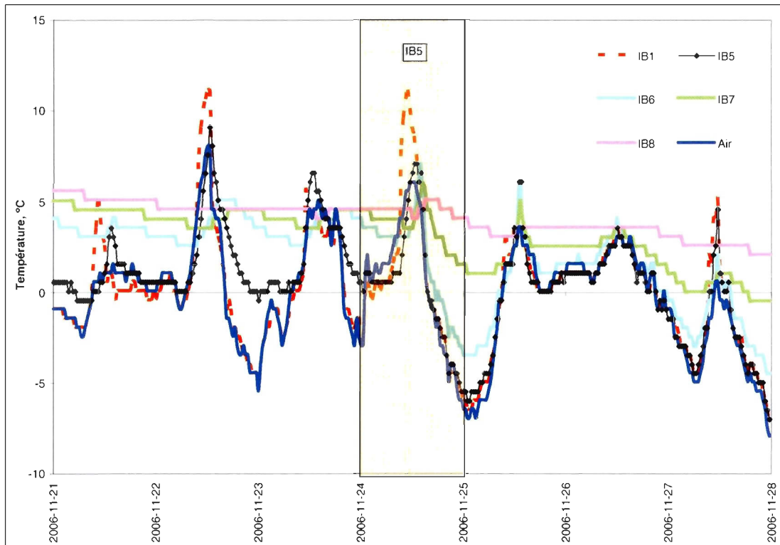
Figure A.25. Signature thermique du recul du 24 novembre impliquant le iB5 de l'unité de silt marin à la station 1.
