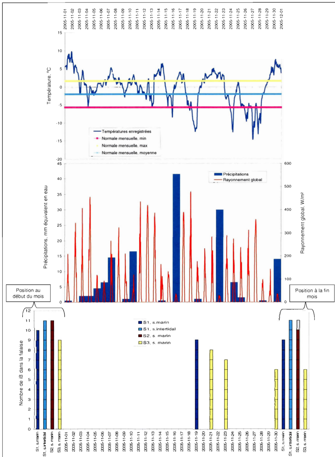
Figure 4.2. Conditions climatiques et reculs des falaises observés au mois de novembre 2005 à Ragueneau.
