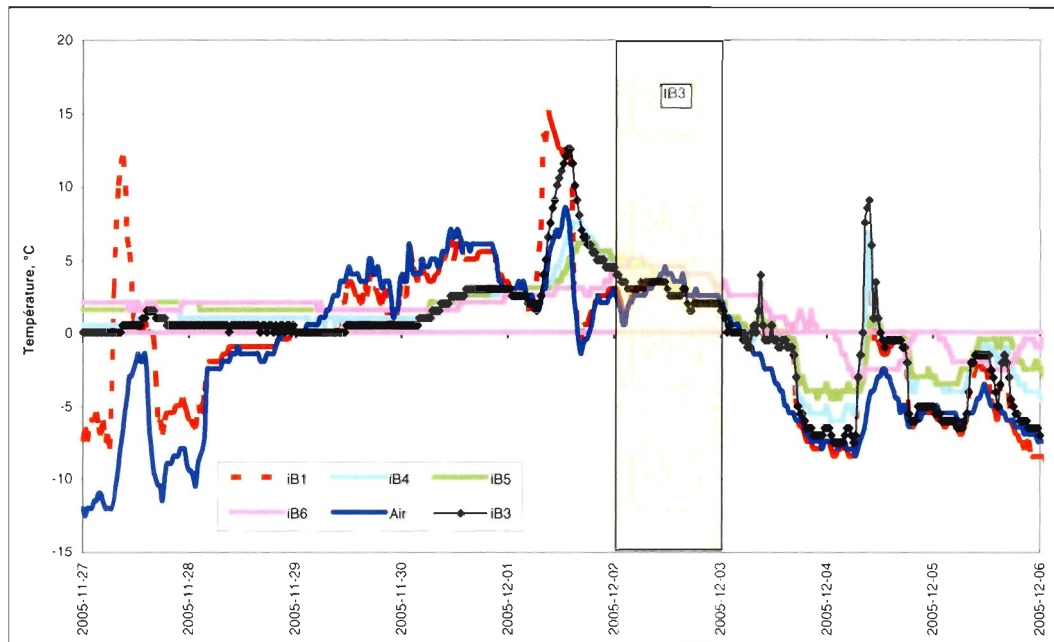
Figure A.7. Signature thermique du recul du 2 décembre 2005 impliquant le iB3 de l'unité de silt marin à la station 2.
