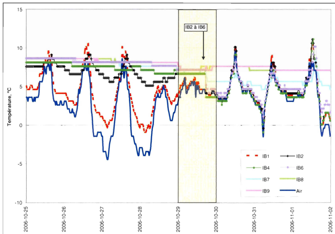
Figure A.20. Signature thermique du recul du 29 octobre 2006 (18 h 00) impliquant le iB2 à iB6 de l'unité de silt intertidal à la station 1.
