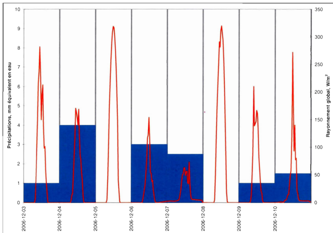
Figure 4.18. Rayonnement global et précipitations enregistrés entre le 4 et 10 décembre 2006 à Ragueneau.
