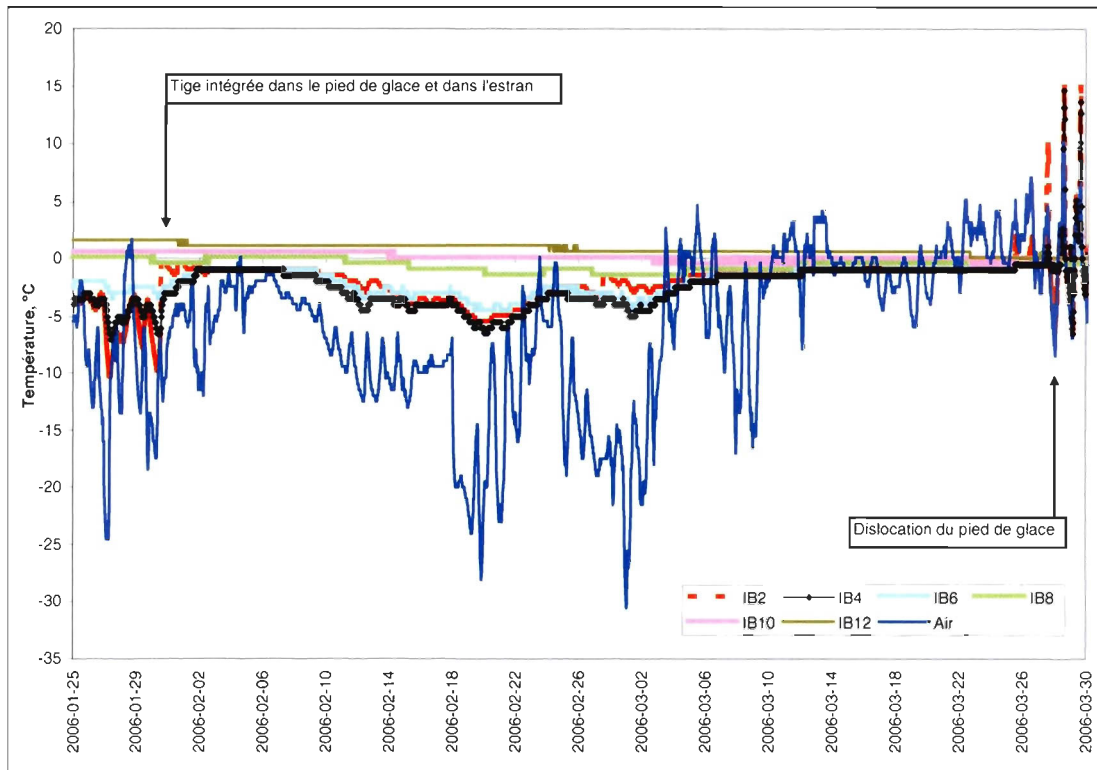
Figure A.10. Stabilité des températures enregistrées par les iButtons suite à la perturbation du 30 janvier de l'unité de silt marin à la station 1.
