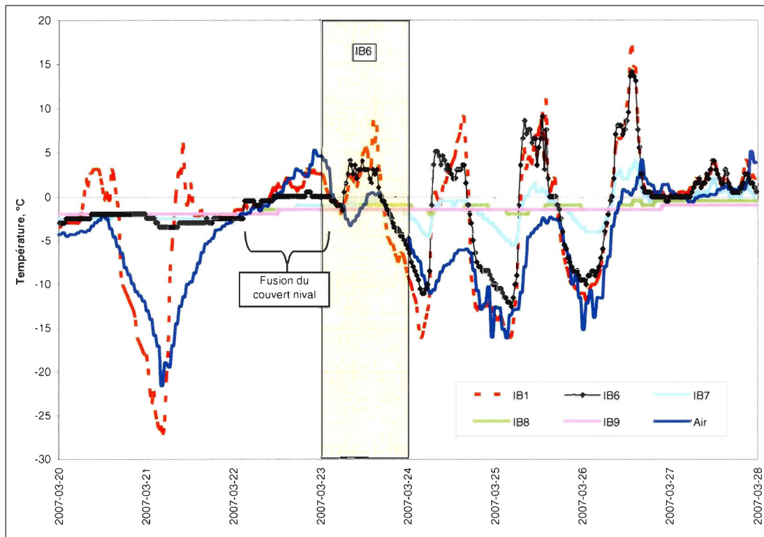
Figure A.32. Signature thermique du recul du 23 mars 2007 impliquant le iB6 de l'unité de silt marin à la station 2.
