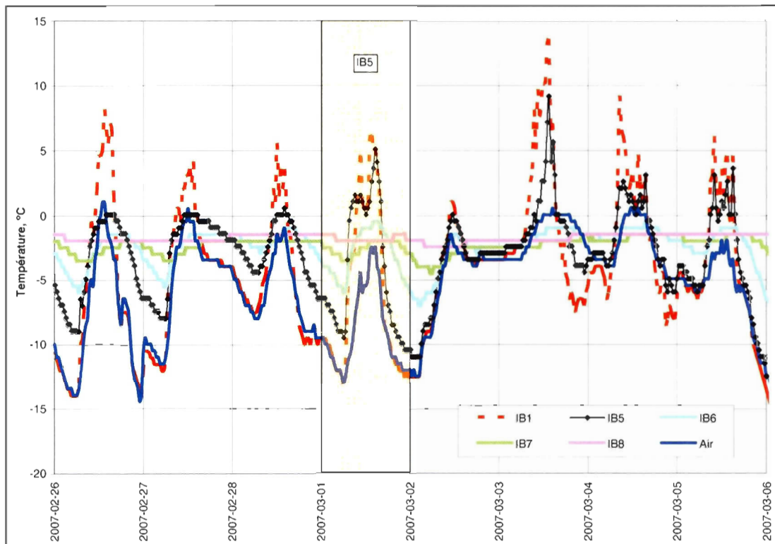
Figure A.31. Signature thermique du recul du 1 er mars 2007 impliquant le iB5 de l'unité de silt marin à la station 2.
