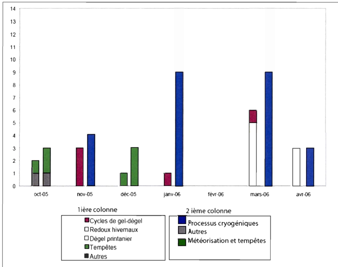
Figure 5.24. Évolution mensuelle des falaises de Ragueneau lors de la saison de suivi 2005-2006.
