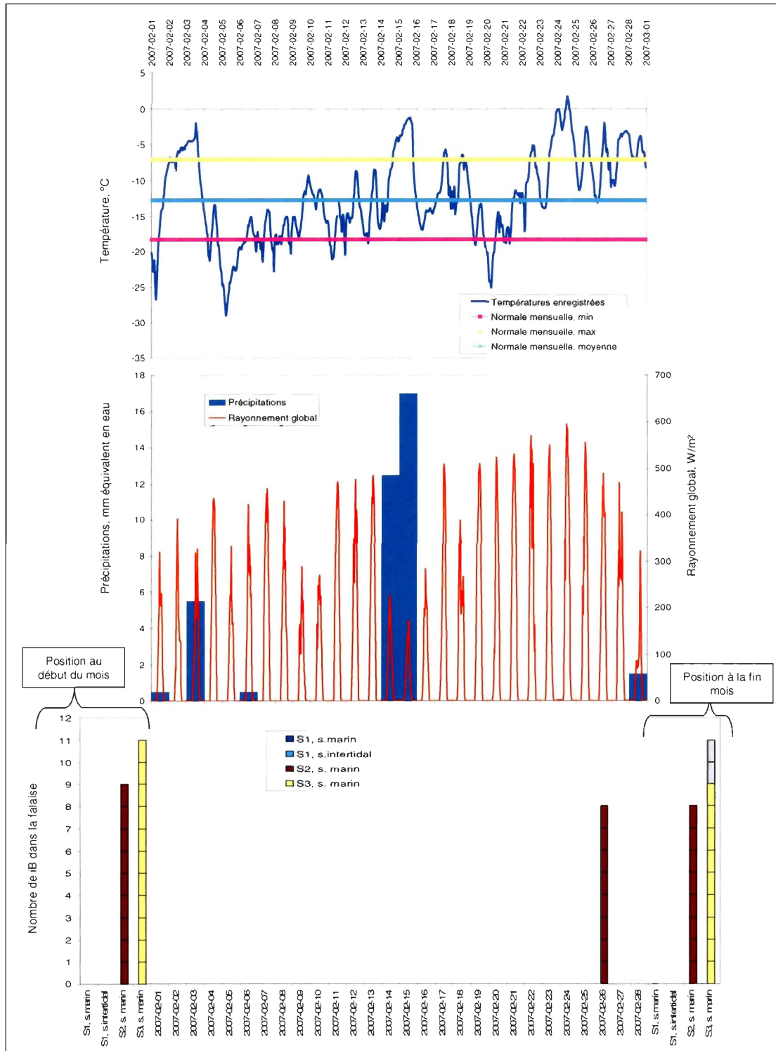
Figure 4.22. Conditions climatiques et reculs des falaises observés au mois de février 2007 à Ragueneau.
