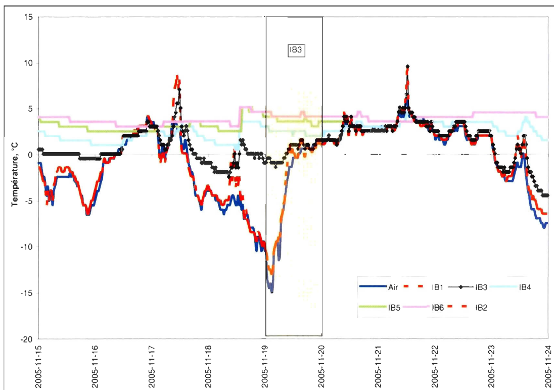
Figure A.3. Signature thermique du recul du 19 novembre 2005 impliquant le iB3 de l'unité de silt marin à la station 1.
