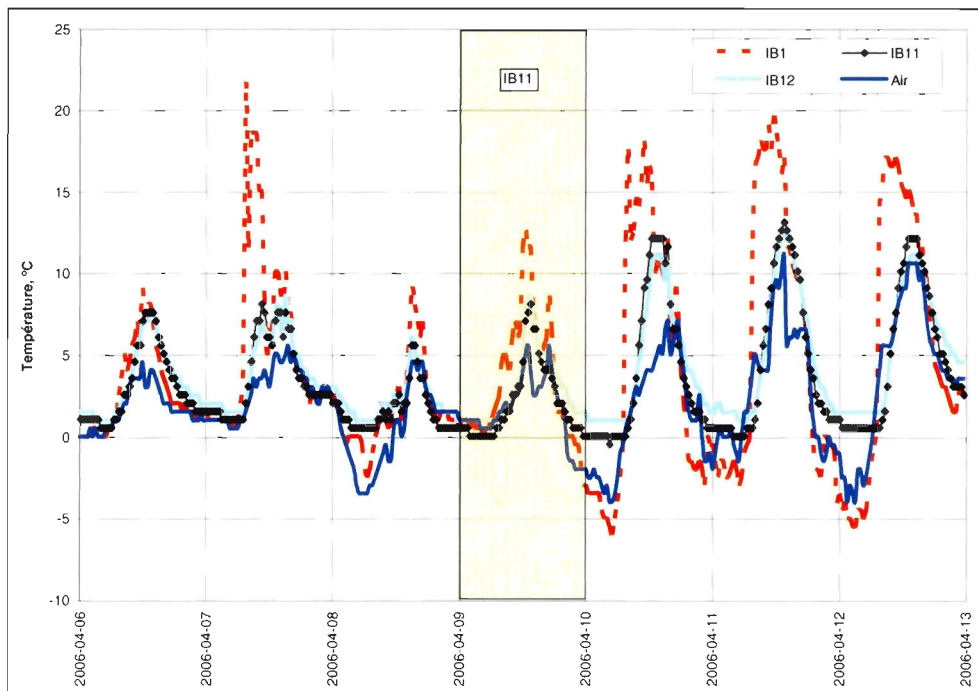
Figure A.18. Signature thermique du recul du 9 avril 2006 impliquant le iB11 de l'unité de silt marin à la station 2.
