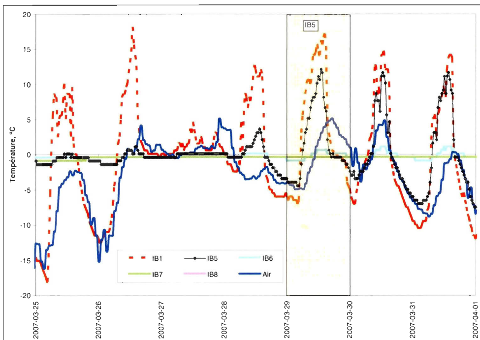
Figure A.35. Signature thermique du recul du 29 mars 2007 impliquant le iB5 de l'unité de silt marin à la station 3.
