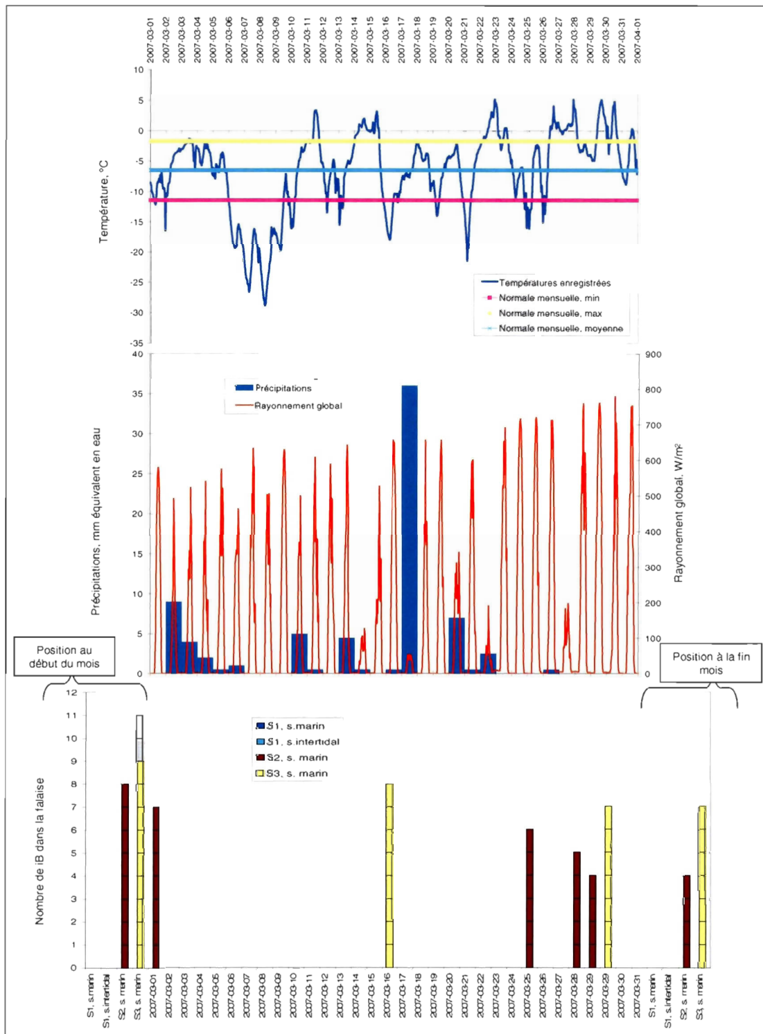
Figure 4.23. Conditions climatiques et reculs des falaises observés au mois de mars 2007 à Ragueneau.
