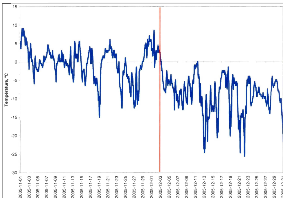
Figure 5.1. Identification du début du régime de températures froides de la saison 2005-2006 le 3 décembre 2005 à Ragueneau.
