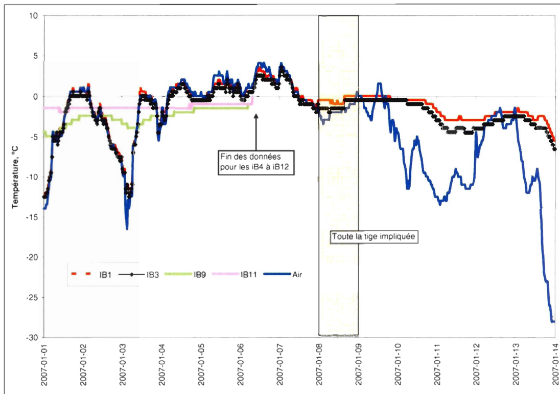
Figure A.29. Signature thermique du recul du 8 janvier 2007 impliquant toute la tige de l'unité de silt intertidal à la station 1.
