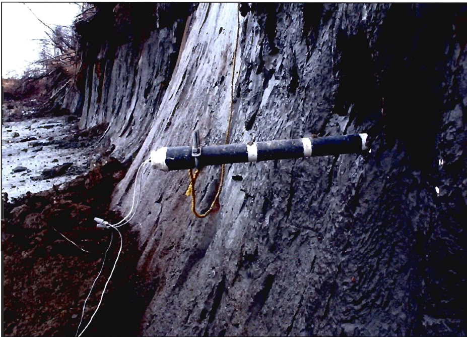
Figure 4.26. Exemple d'un iButton à la limite externe de la falaise engendrant des difficultés dans l'analyse des signatures thermiques à la station 1.
