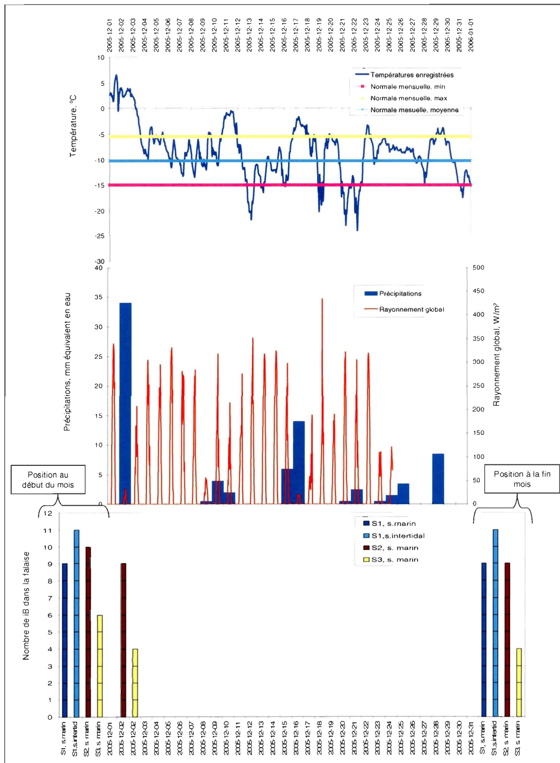
Figure 4.4. Conditions climatiques et reculs des falaises observés au mois de décembre 2005 à Ragueneau.
