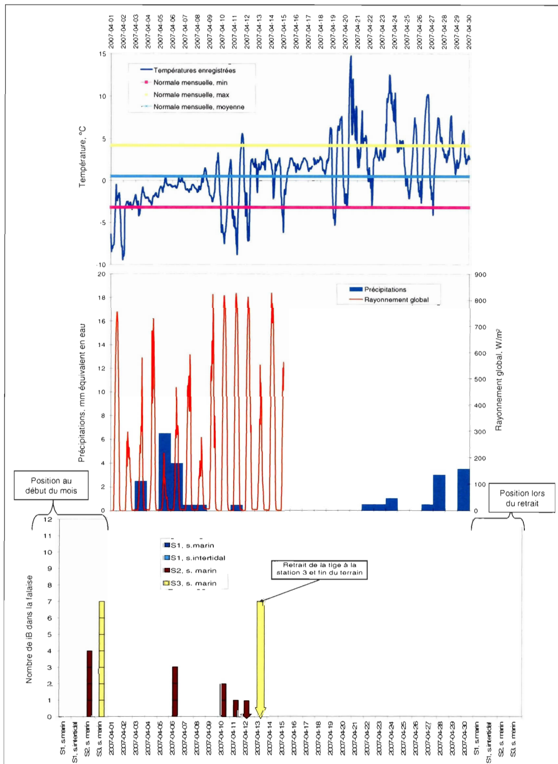
Figure 4.24. Conditions climatiques et reculs des falaises observés au mois d'avril 2007 à Ragueneau.
