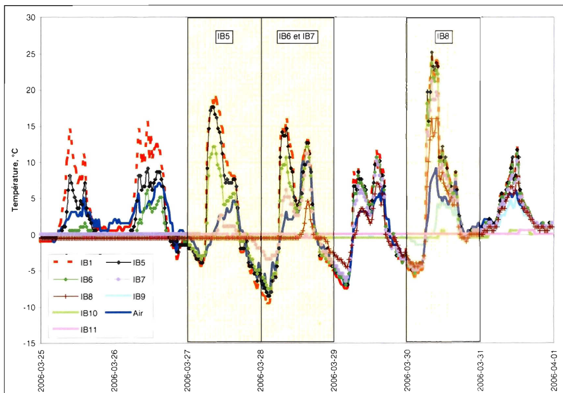
Figure A.13. Signature thermique des reculs du 27, 28 et du 30 mars 2006 impliquant les iB5 à iB8 de l'unité de silt marin à la station 2.
