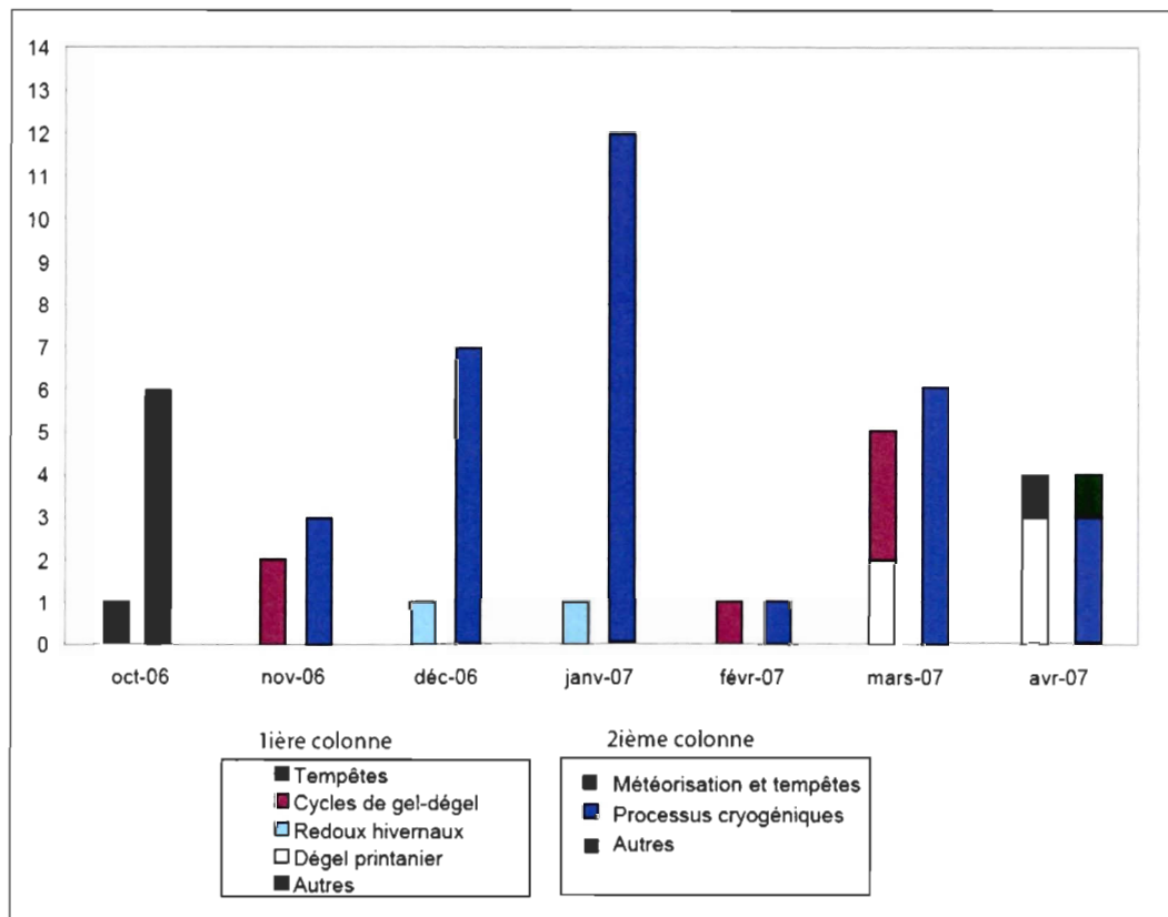
Figure 5.25. Évolution mensuelle des falaises de Ragueneau lors de la saison de suivi 2006-2007.
