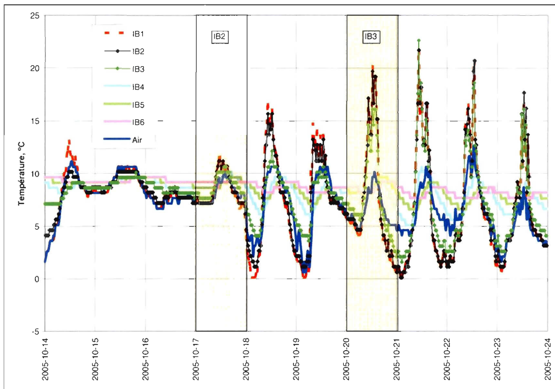
Figure A.2. Signature thermique des reculs du 17 et du 20 octobre 2005 impliquant les iB2 et iB3 de l'unité de silt marin à la station 3.
