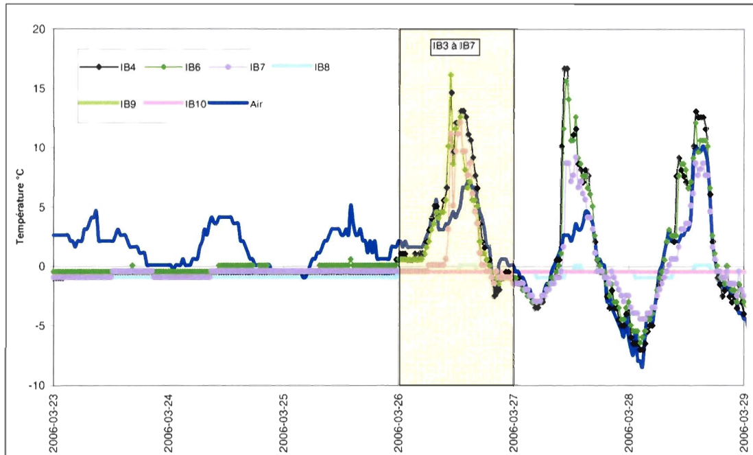
Figure A.12. Signature thermique du recul du 26 mars 2006 impliquant les iB3 à iB7 de l'unité de silt intertidal à la station 1.
