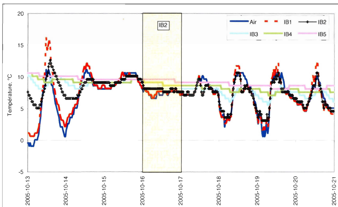
Figure A.1. Signature thermique du recul du 16 octobre 2005 impliquant le iB2 de l'unité de silt marin à la station 1.
