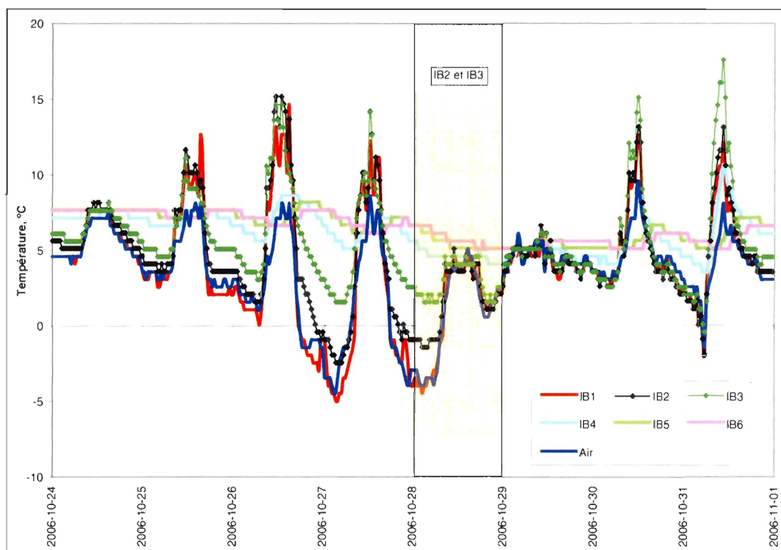
Figure A.19. Signature thermique du recul du 28 octobre 2006 impliquant le iB2 et le iB3 de l'unité de silt marin à la station 2.
