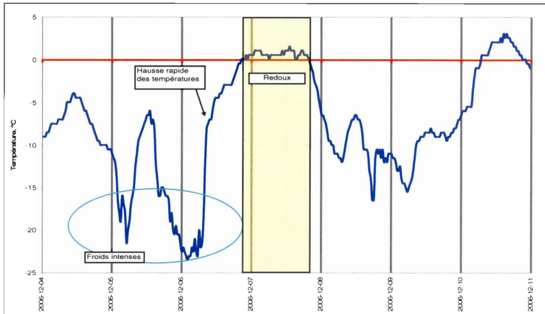
Figure 4.17. Températures de l'air enregistrées entre le 4 et 10 décembre 2006 à Ragueneau.
