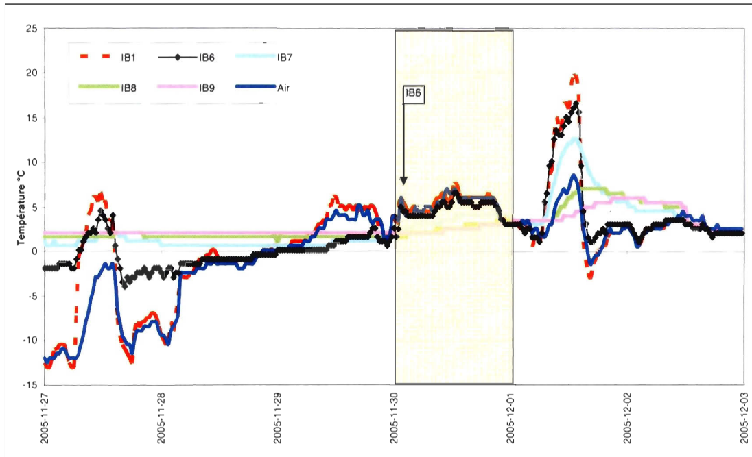
Figure A.6. Signature thermique du recul du 30 novembre 2005 impliquant le iB6 de l'unité de silt marin à la station 3.
