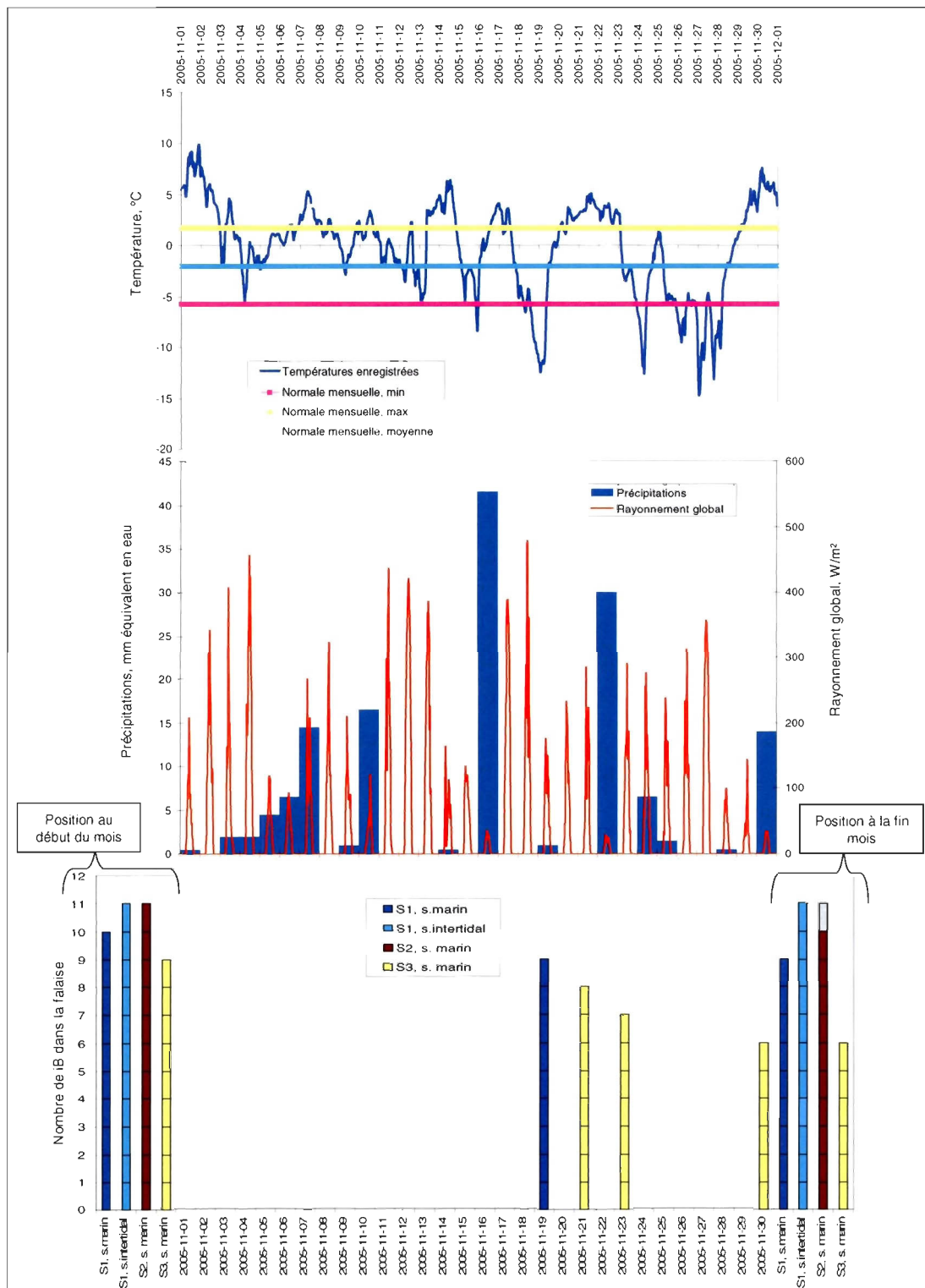
Figure 2.6. Exemple d'une figure synthèse mensuelle : novembre 2005.
