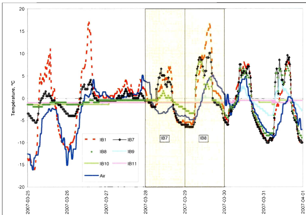
Figure A.34. Signature thermique des reculs du 28 et 29 mars 2007 impliquant les iB7 et iB8 de l'unité de silt marin à la station 2.
