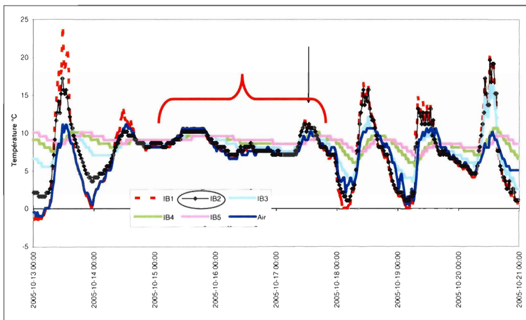
Figure 4.25. Isothermie des températures observées les 15 et 16 octobre 2006 et signature du recul de la falaise du 17 octobre impliquant le iB2 de l'unité de silt marin à la station 3.
