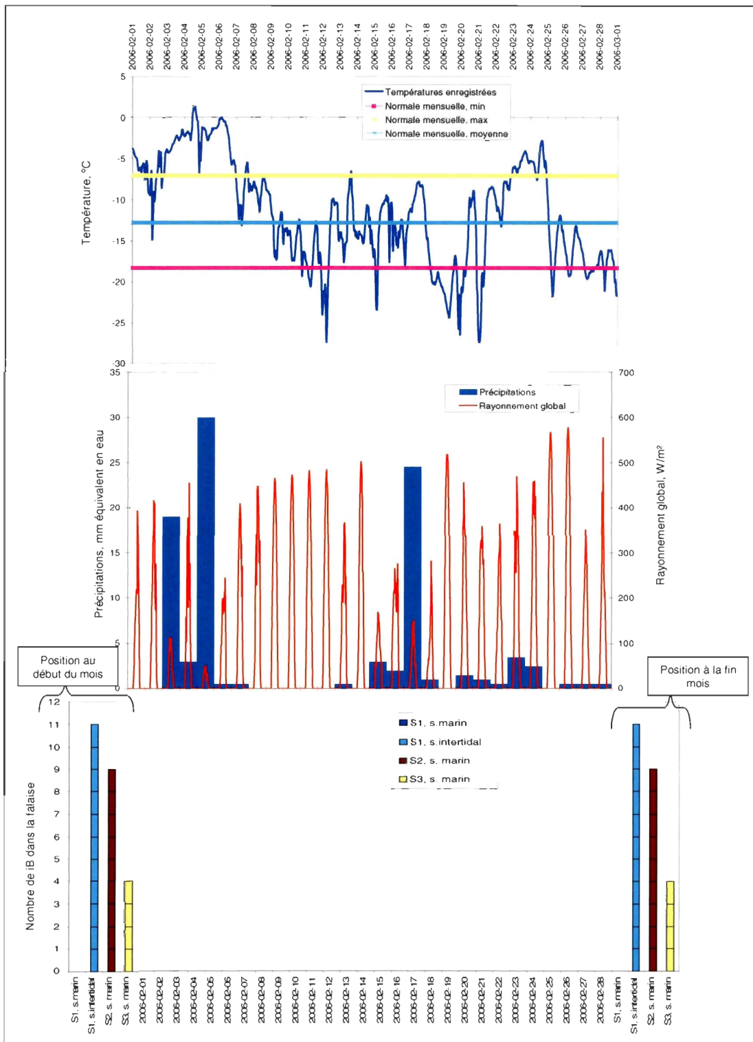
Figure 4.8. Conditions climatiques et reculs des falaises observés au mois de février 2006 à Ragueneau.
