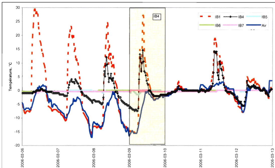
Figure A.11. Signature thermique du recul du 9 mars 2006 impliquant le iB4 de l'unité de silt marin à la station 2.
