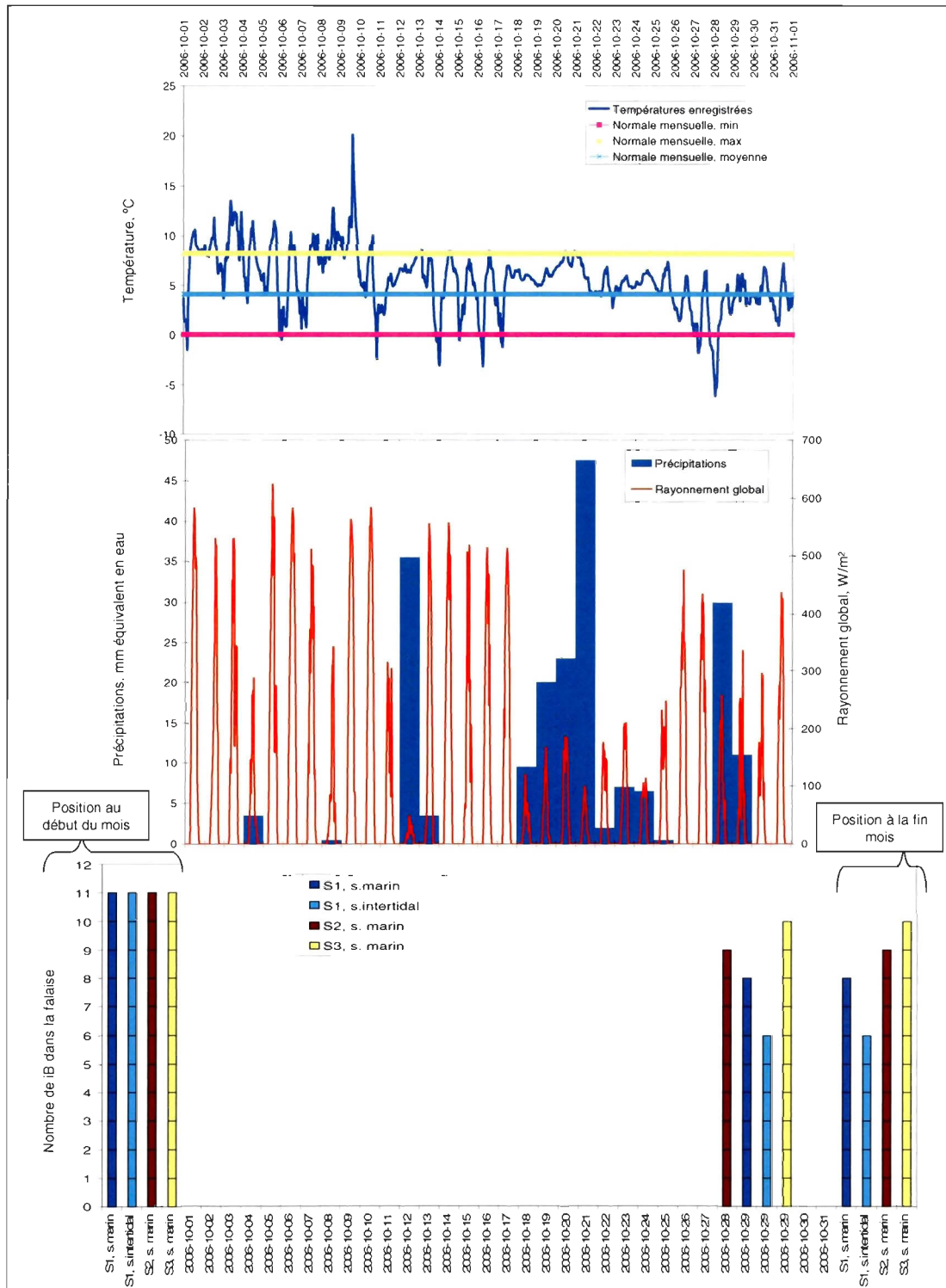
Figure 4.13. Conditions climatiques et reculs des falaises observés au mois d'octobre 2006 à Ragueneau.
