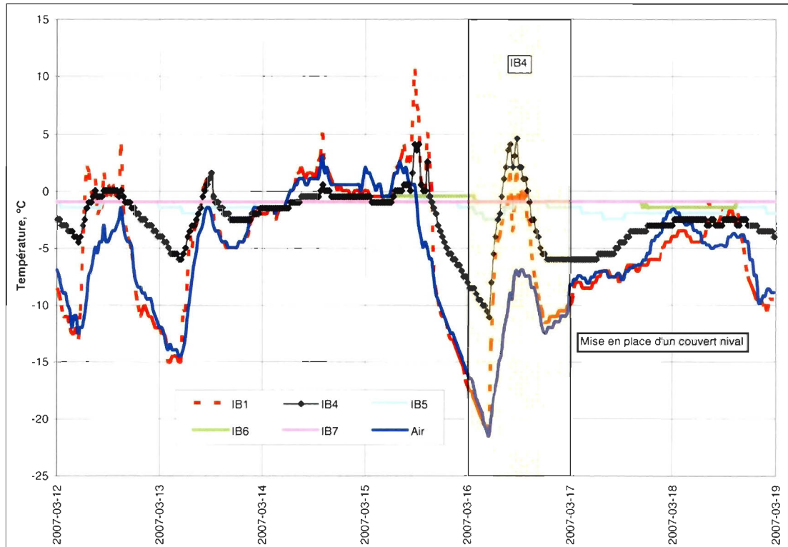
Figure A.33. Signature thermique du recul du 16 mars 2007 impliquant le iB4 de l'unité de silt marin à la station 3.
