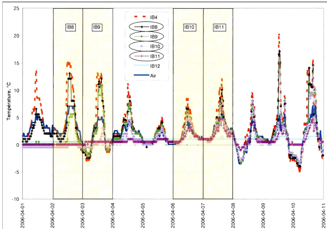
Figure A.16. Signature thermique des reculs du 2, 3, 6 et 7 avril 2006 impliquant les iB8 à iB11 de l'unité de silt intertidal de la station 1.
