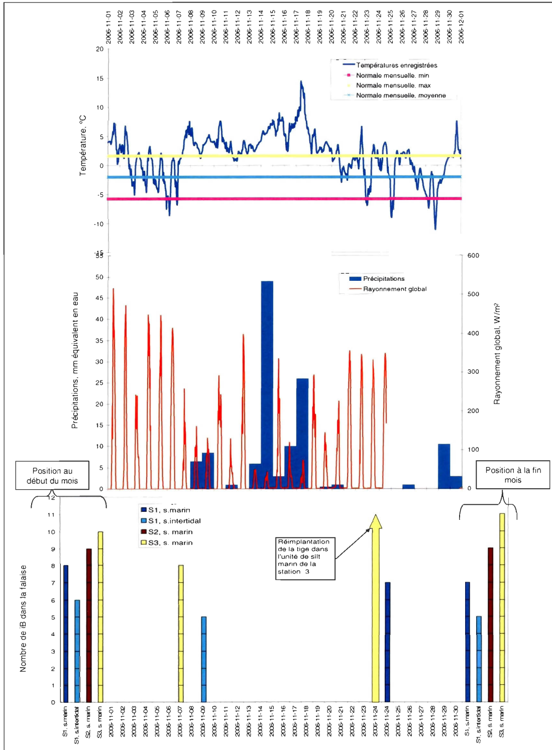
Figure 4.14. Conditions climatiques et reculs des falaises observés au mois de novembre 2006 à Ragueneau.
