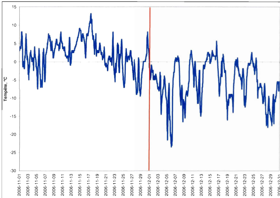
Figure 5.2. Identification du début du régime de température froide de la saison 2006-2007 le 1 er décembre 2006 à Ragueneau.
