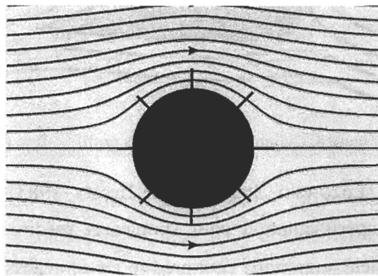
Figure 7. Les lignes de courant de l'écoulement potentiel autour d'un cylindre circulaire discrétisé par des panneaux.
