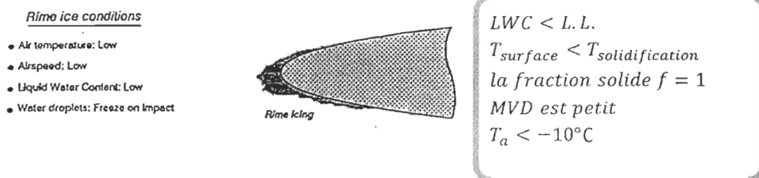
Figure 5. Le régime sec (le givre)
