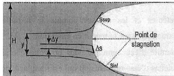
Figure 3. Définition de l'efficacité de collection
