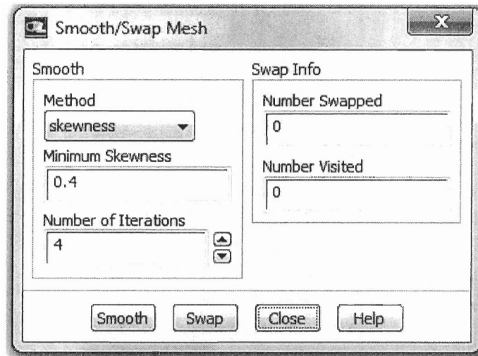
Figure 37: Lissage du maillage par Fluent
