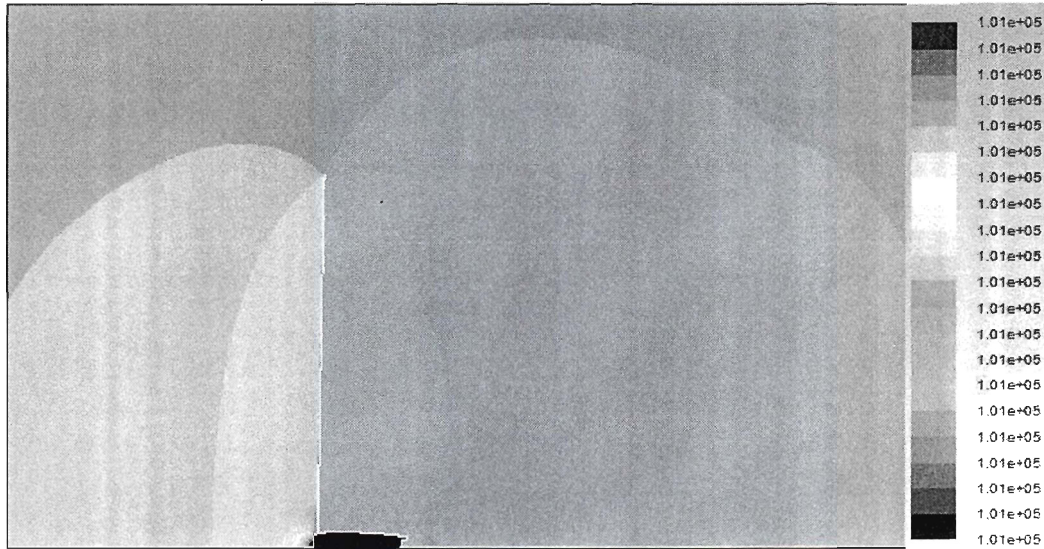
Figure 36 : Allure des contours de la pression pour une simulation réalisée avec le modèle de turbulence SST k-\omega , une vitesse du vent de 10m/s et une vitesse de rotation de 13 tours/minutes
