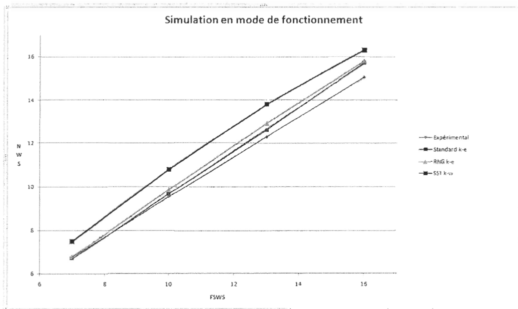
Figure 28: Comparaison des résultats de simulation des divers modes de turbulence et des résultats expérimentaux.
