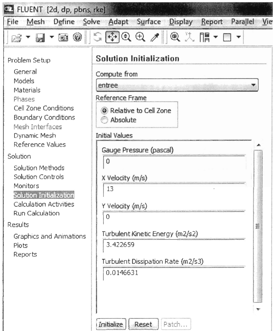
Figure 50: Initialisation des calculs de Fluent
