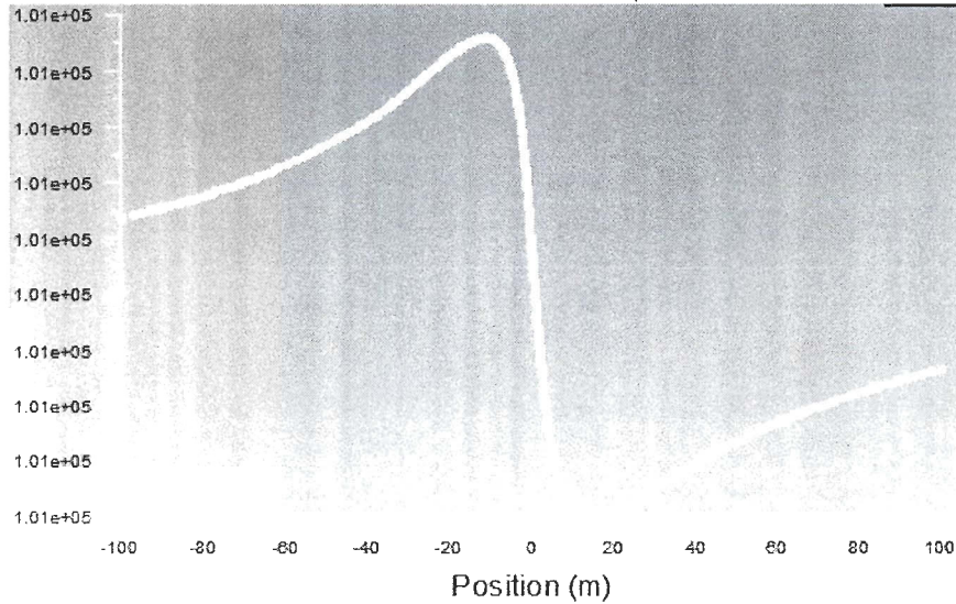
Figure 39 : Allure de la pression sur une ligne passant à 20m au-dessus de la nacelle pour une simulation réalisée avec le modèle de turbulence k-\omega SST, une vitesse du vent de 10m/s et une vitesse de rotation de 13 tours/minutes
