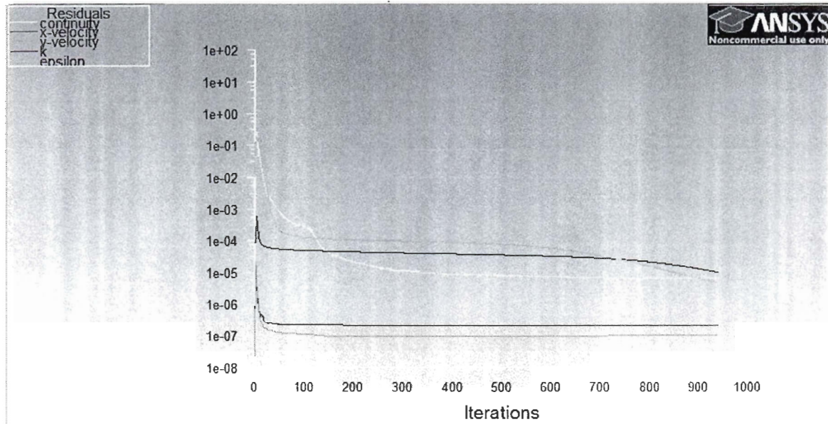
Figure 13: Observations des courbes des résidus pour la continuité, la vitesse et la turbulence pour le modèle k- \epsilon STANDARD pour une vitesse d'entrée de 16m/s
