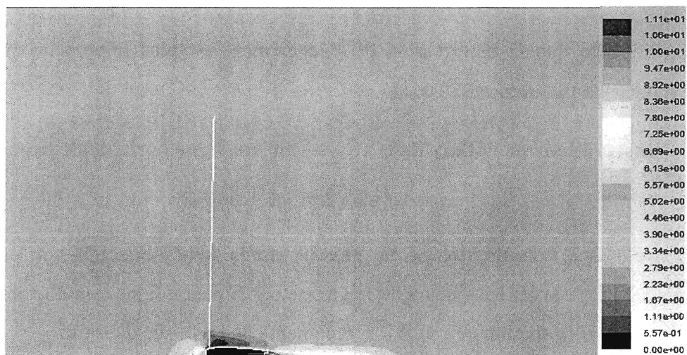
Figure 41 : Allure des contours de la vitesse pour une simulation réalisée avec le modèle de turbulence RNG k-\varepsilon , une vitesse du vent de 10m/s et une vitesse de rotation de 13 tours/minutes
