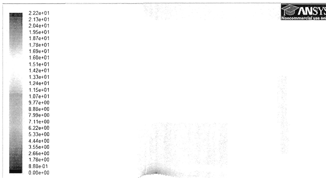
Figure 22: Représentation des contours de la vitesse pour une vitesse d'entrée de 16m/s pour le modèle k-ε STANDARD
