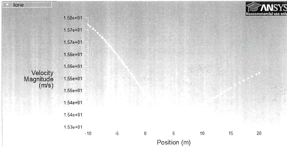
Figure 25: Allure de la vitesse à la traversée du rotor pour une vitesse d'entrée de 16m/s à 15m de hauteur pour le modèle k- \epsilon STANDARD
