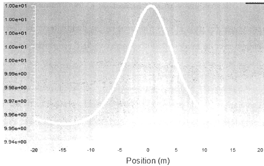
Figure 44 : Allure de la vitesse sur une ligne passant à 20m au-dessus de la nacelle pour une simulation réalisée avec le modèle de turbulence RNG k-\epsilon , une vitesse du vent de 10m/s et une vitesse de rotation de 13 tours/minutes
