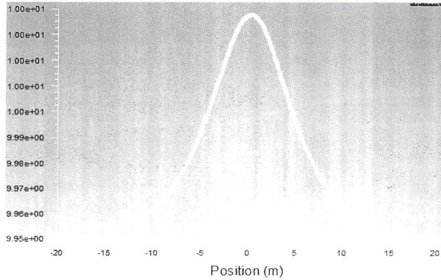
Figure 43 : Allure de la vitesse sur une ligne passant à 20m au-dessus de la nacelle pour une simulation réalisée avec le modèle Standard k-\epsilon , une vitesse du vent de 10m/s et une vitesse de rotation de 13 tours/minutes
