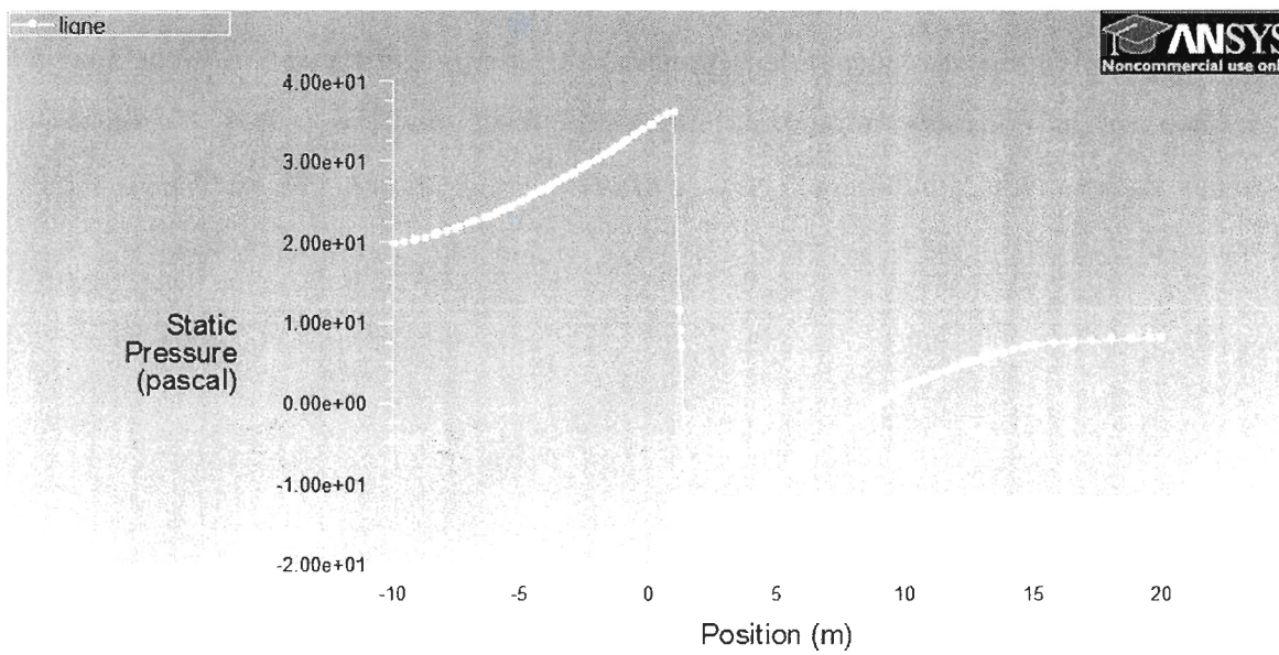
Figure 20 : Allure de la pression à la traversée du rotor pour une vitesse d'entrée de 16m/s à 15m de hauteur pour le modèle k- \epsilon RNG
