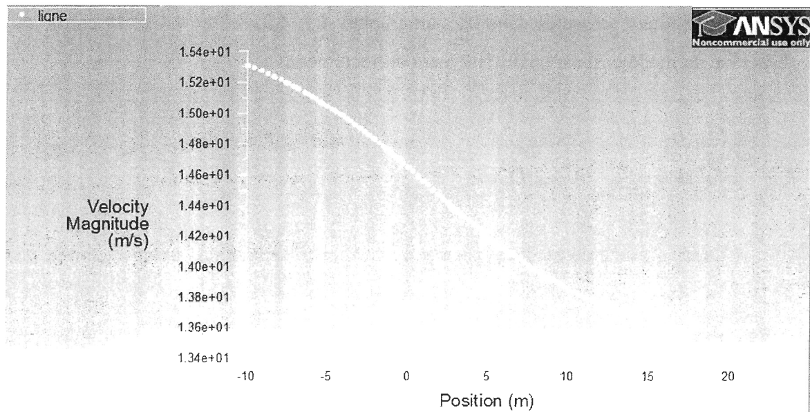
Figure 27: Allure de la vitesse à la traversée du rotor pour une vitesse d'entrée de 16m/s à 15m de hauteur pour le modèle k- \omega SST
