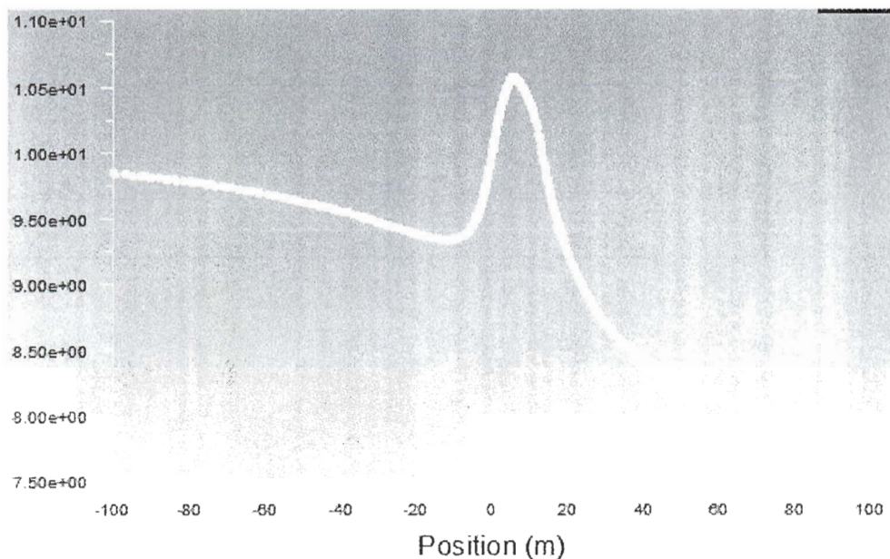
Figure 45 : Allure de la vitesse sur une ligne passant à 20m au-dessus de la nacelle pour une simulation réalisée avec le modèle de turbulence k-\omega SST, une vitesse du vent de 10m/s et une vitesse de rotation de 13 tours/minutes
