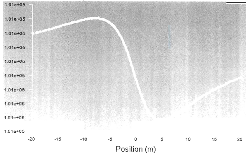
Figure 37 : Allure de la pression sur une ligne passant à 20m au-dessus de la nacelle pour une simulation réalisée avec le modèle de turbulence Standard k- \epsilon , une vitesse du vent de 10m/s et une vitesse de rotation de 13 tours/minutes
