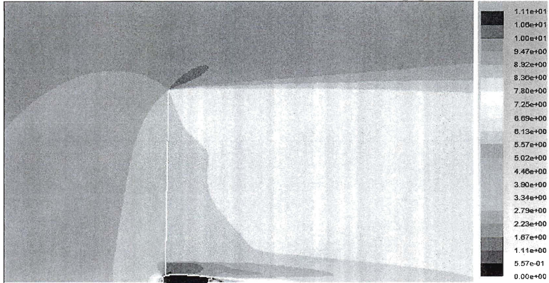
Figure 42 : Allure des contours de la vitesse pour une simulation réalisée avec le modèle de turbulence SST k-\omega , une vitesse du vent de 10m/s et une vitesse de rotation de 13 tours/minute
