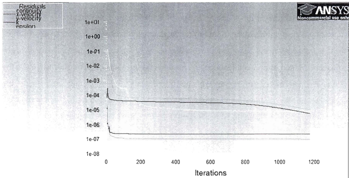
Figure 14: Observations des courbes des résidus pour la continuité, la vitesse et la turbulence pour le modèle k- \epsilon RNG pour une vitesse d'entrée de 16m/s
