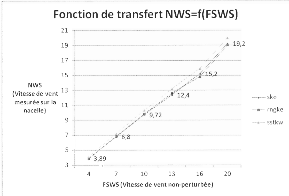
Figure 46 : Détermination numérique de la relation entre la vitesse du vent sur la nacelle en fonction de la vitesse du vent non perturbée
