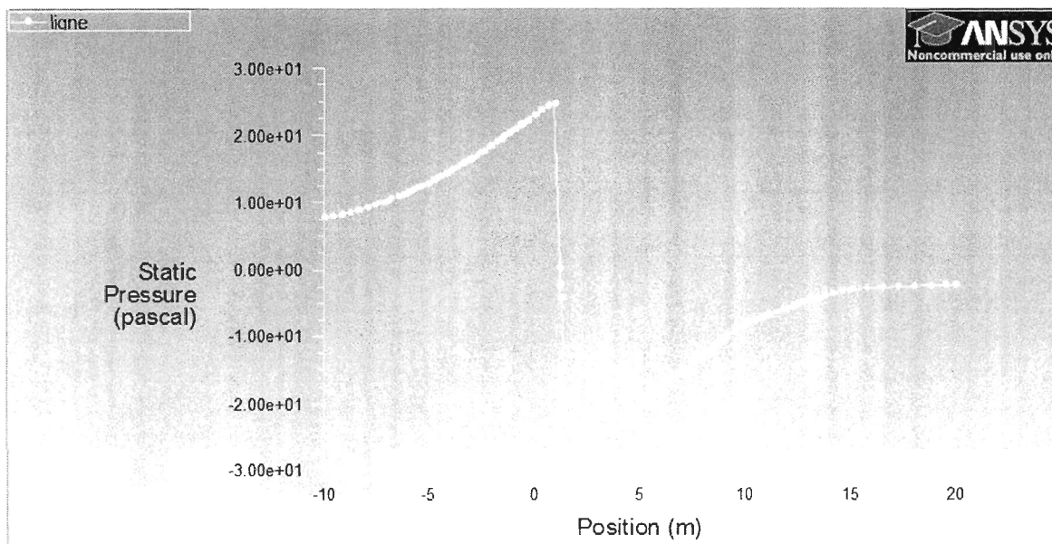
Figure 19 : Allure de la pression à la traversée du rotor pour une vitesse d'entrée de 16m/s à 15m de hauteur pour le modèle k- \epsilon STANDARD
