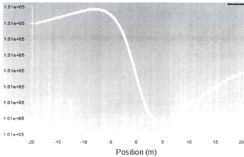
Figure 38 : Allure de la pression sur une ligne passant à 20m au-dessus de la nacelle pour une simulation réalisée avec le modèle de turbulence RNG k- \epsilon , une vitesse du vent de 10m/s et une vitesse de rotation de 13 tours/minutes
