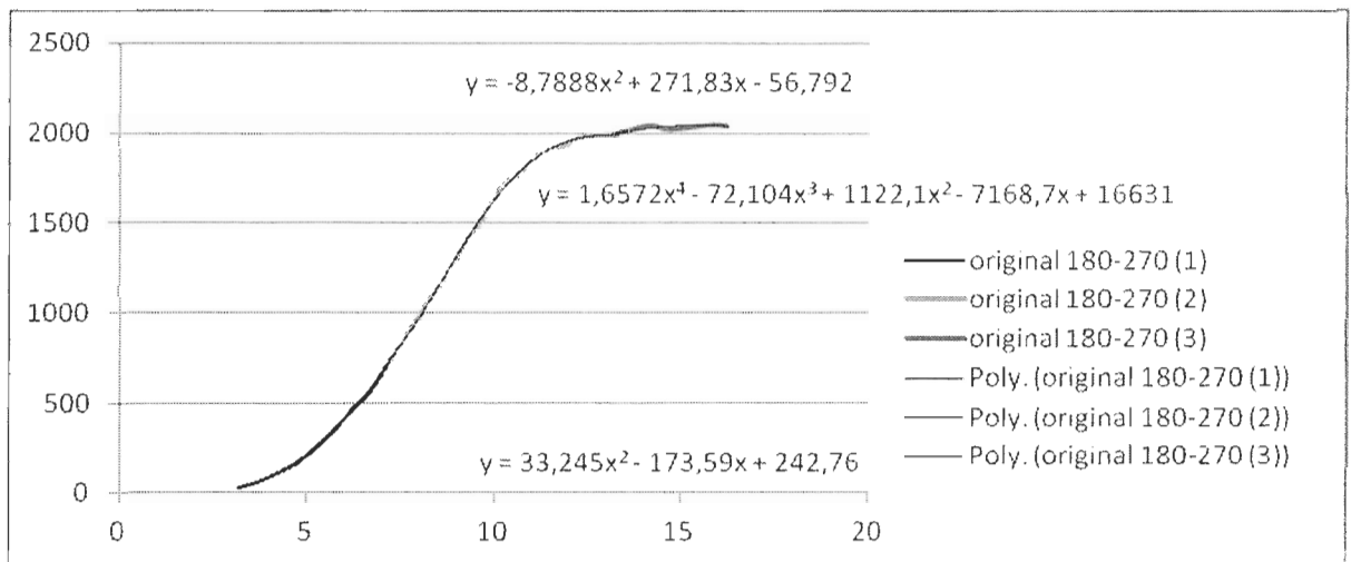
Figure 30 : Détermination de l'équation de la courbe de puissance mesurée dans le secteur 270-360
