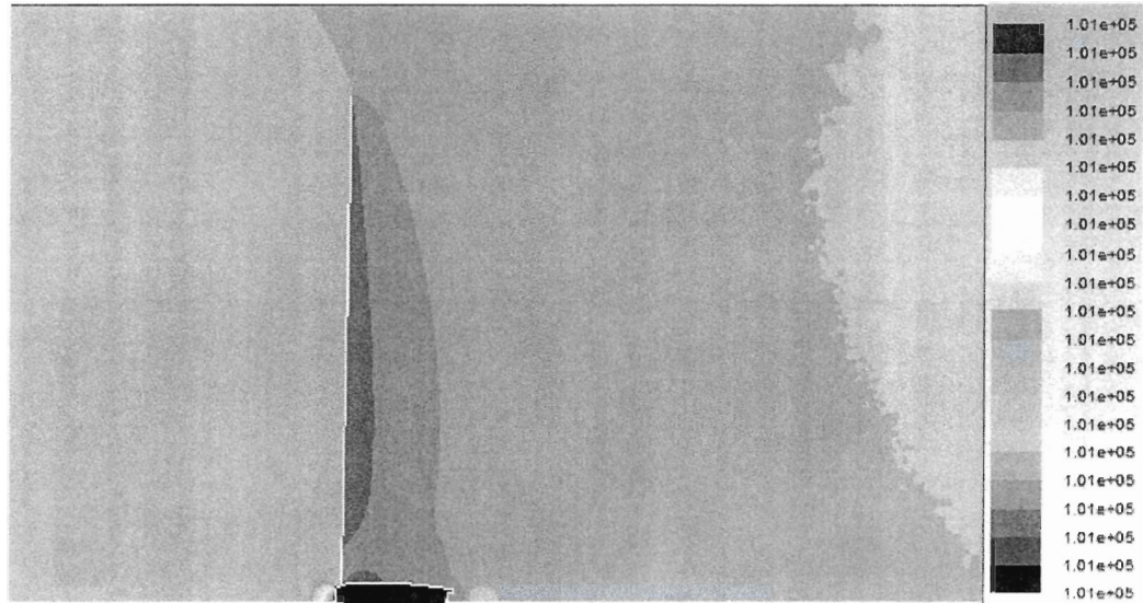
Figure 34 : Allure des contours de la pression pour une simulation réalisée avec le modèle de turbulence Standard k-\epsilon , une vitesse du vent de 10m/s et une vitesse de rotation de 13 tours/minutes
