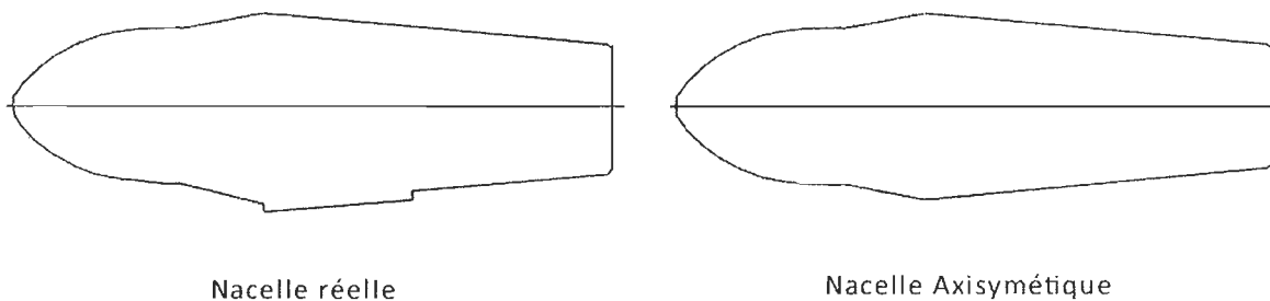
Figure 8 : Profil transversal de la nacelle dans les cas réel et axisymétrique
