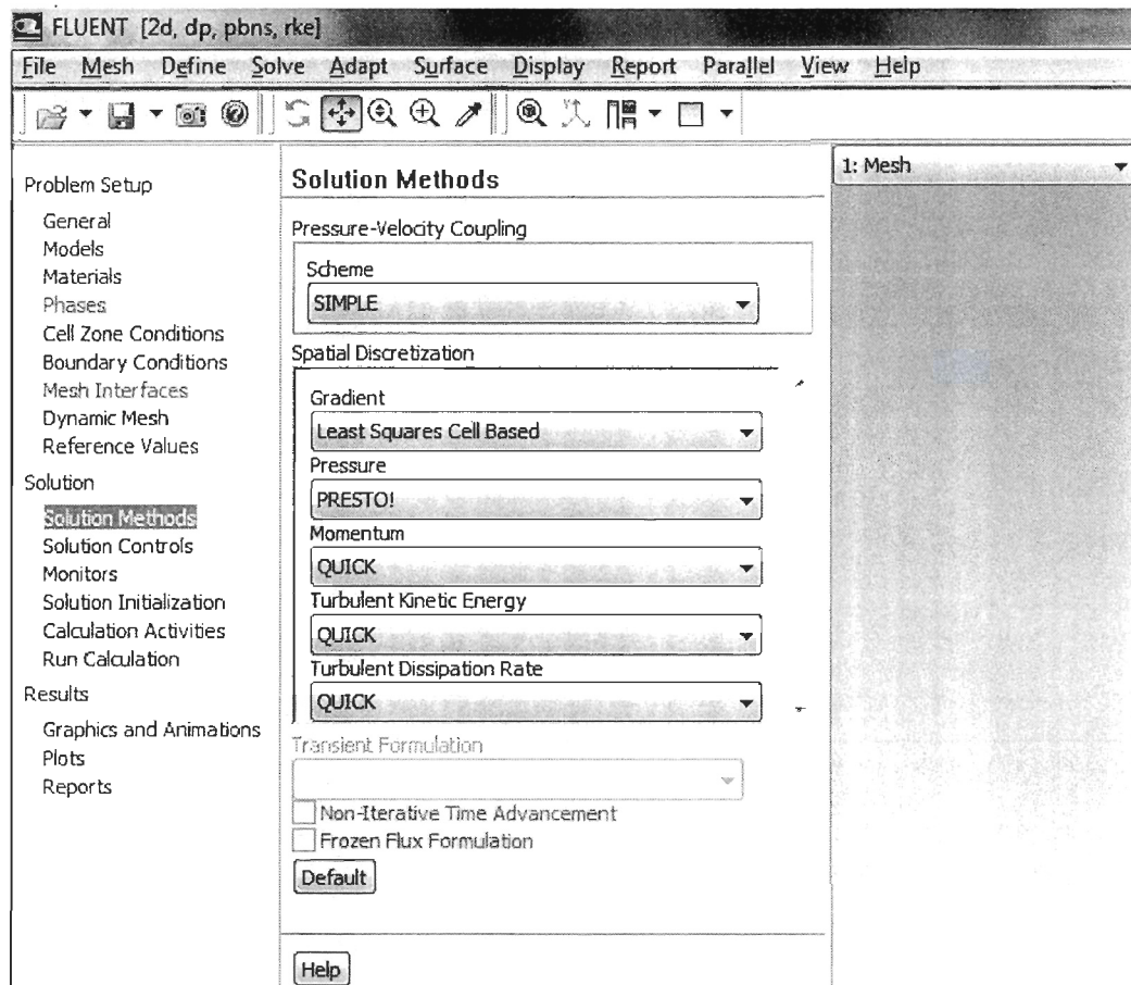
Figure 47: Choix des algorithmes de calculs de Fluent
