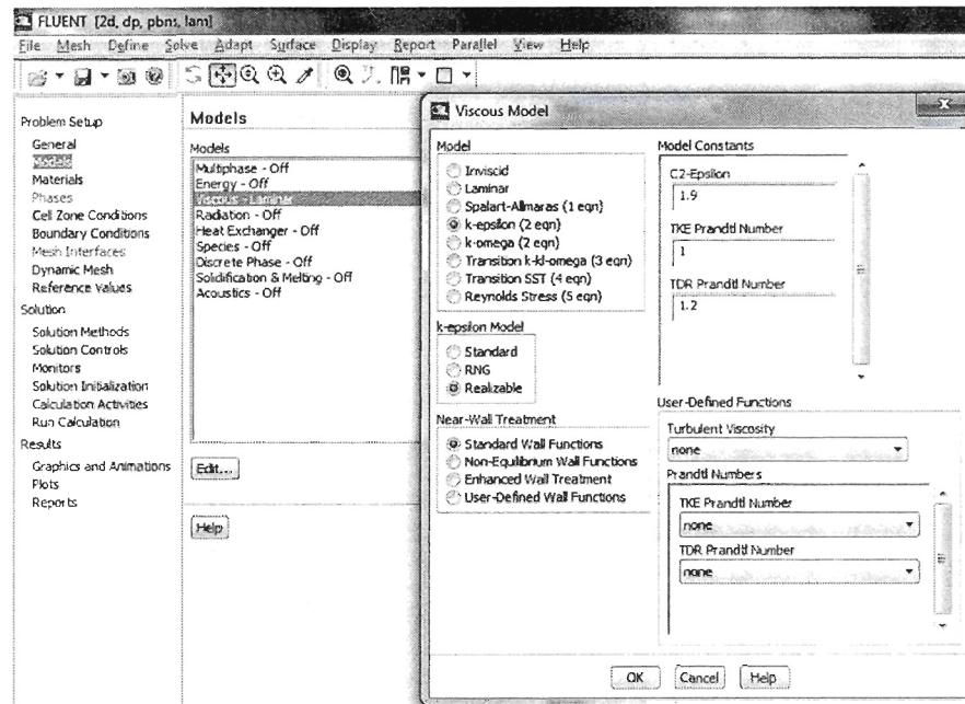
Figure 42: Choix du modèle de turbulence k-\epsilon Realizable dans Fluent
