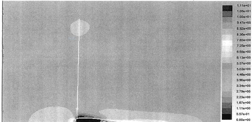
Figure 40 : Allure des contours de la vitesse pour une simulation réalisée avec le modèle de turbulence Standard k-\varepsilon , une vitesse du vent de 10m/s et une vitesse de rotation de 13 tours/minutes
