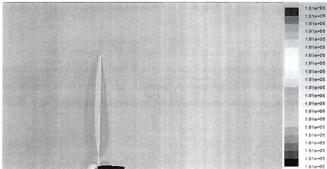
Figure 35 : Allure des contours de la pression pour une simulation réalisée avec le modèle de turbulence RNG k-\epsilon , une vitesse du vent de 10m/s et une vitesse de rotation de 13 tours/minutes
