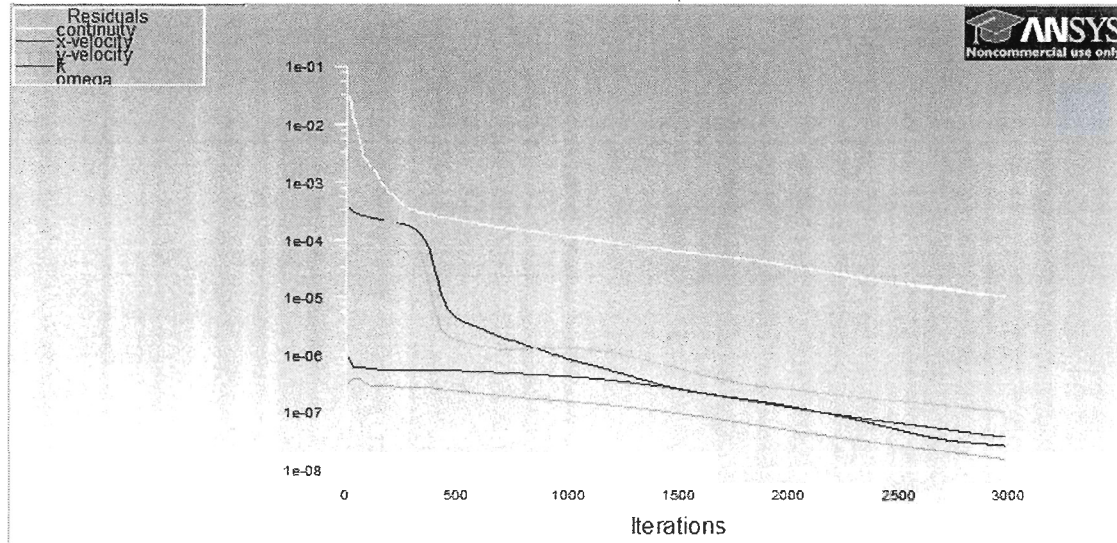
Figure 15: Observations des courbes des résidus pour la continuité, la vitesse et la turbulence pour le modèle k-\omega SST pour une vitesse d'entrée de 16m/s
