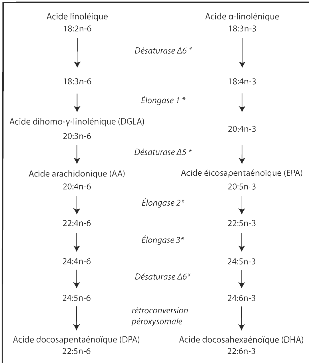
Figure 3 Voies de biosynthèse des acides gras essentiels des séries n-3 et n-6 chez le poisson. * réactions ayant lieu dans les microsomes.
