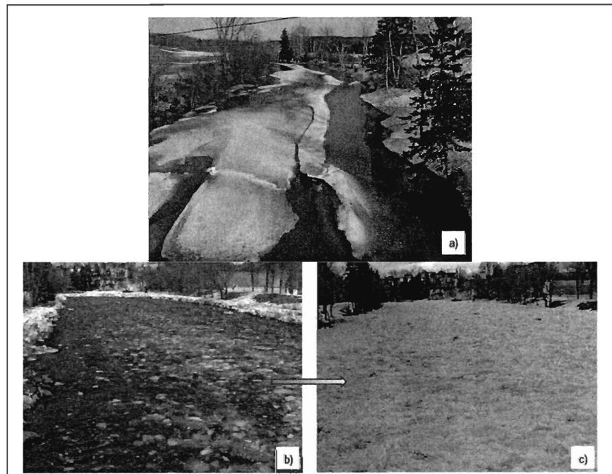
Figure 1.9 : Débâcle thermique versus débâcle mécanique (a), où le couvert fond sous l'effet des rayonnement solaire ; (b) où la pression exercée par une augmentation rapide du débit cause le fractionnement du couvert de glace en blocs pouvant mener à un embâcle (c)
