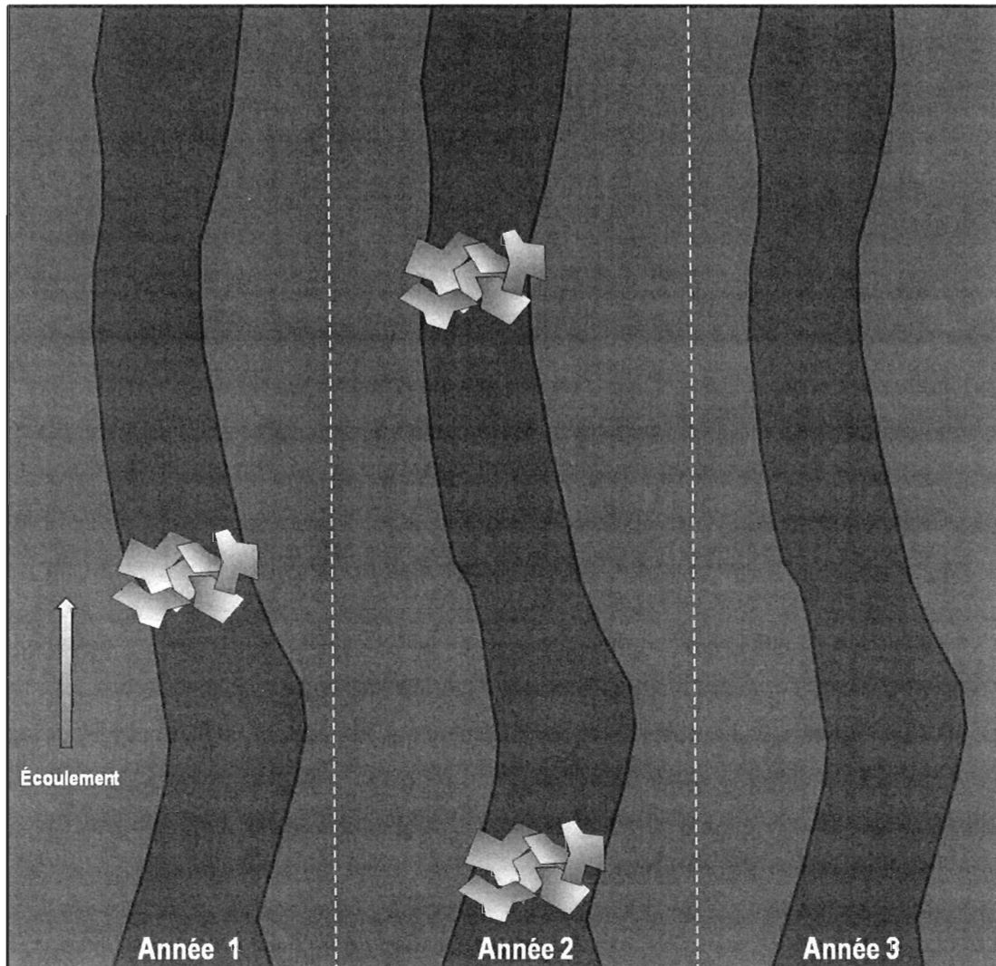
Figure 1.1 : Schématisation de l'irrégularité de la dynamique spatio-temporelle de la formation d'embâcle pour un même tronçon de rivière © Suzan MacNider Taylor, 2010
