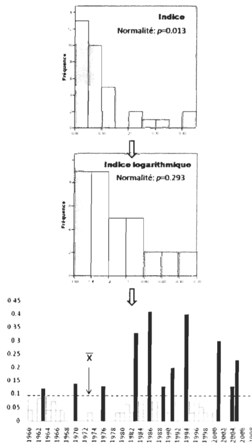
Figure 1.18 : Procédure d'identification d'événements d'embâcles
