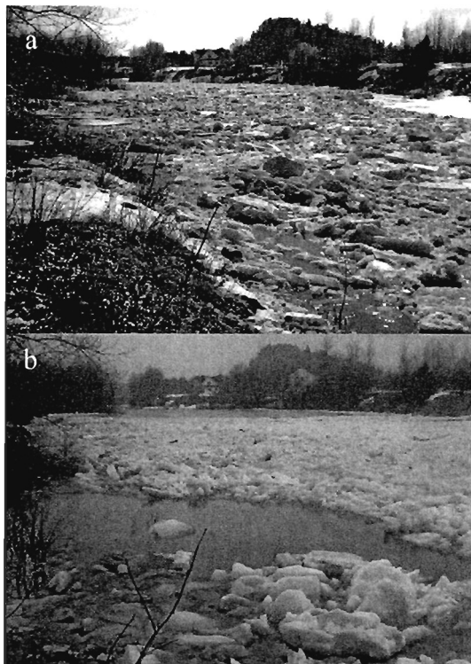
Figure 1.3. a) Embâcle de glace b) Inondation causée par un embâcle. Rivière Ouelle, le 12 avril 2009 Les 2 photos : ©Suzan MacNider Taylor, 2010
